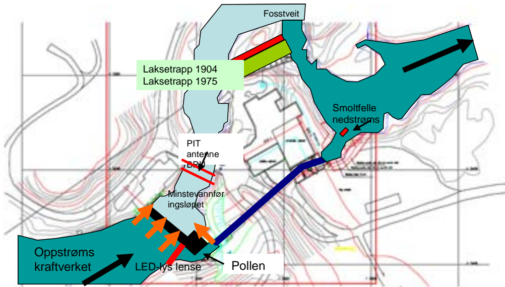
Figur 3. Illustrasjon av vannløpene ved Fossstveit kraftverk. Damkrona er markert sort. De fire oransje pilene markerer henholdsvis laksetrapp, smoltoverløpet, renseløpet og badeland. Badeland er da nærmest rørgata til turbinen og inni selve pollen. Denne rørgata er vist med mørk blå farge. PIT-merka fisk som nedvandrer til minstevannføringsløpet kan gjenfanges i PIT-BRU og må nedvandre enten via laksetrappa eller via fossen Fossstveit før de igjen er i Storelva. Dette var nedvandningsruta før kraftverket ble reetablert i 2008. Plasseringen av LED-lyset er vist med rød strek.
