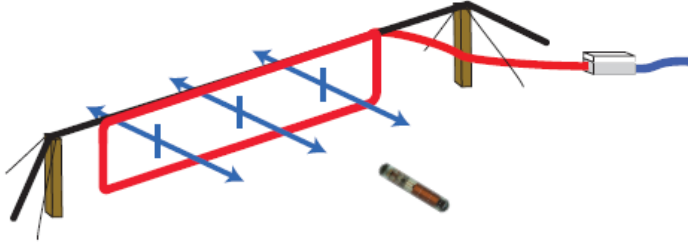
Figur 5. Illustrasjon av antennesløyfe. Illustrasjonen er hentet fra ( http://www.oregonrfid.biz )
