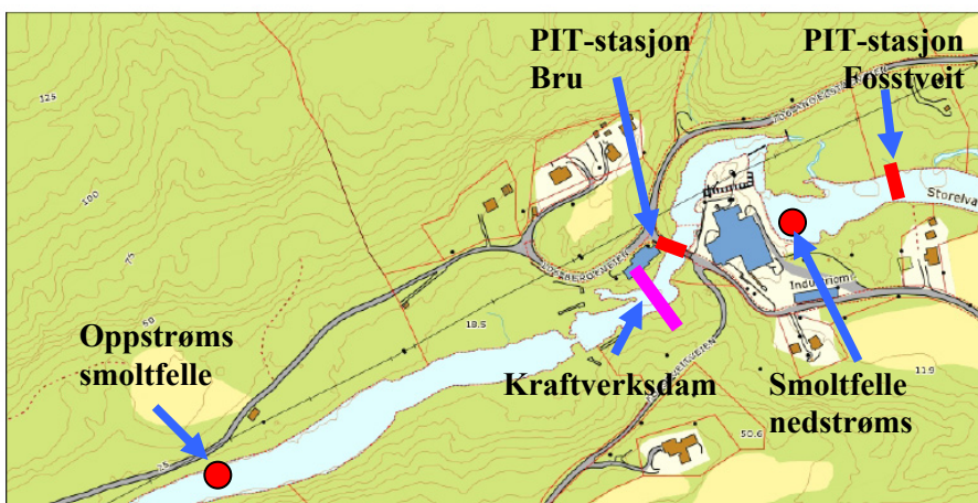
Figur 6. Plassering av de ulike merke- og gjenfangststasjonene omkring Fossveit kraftverk. Smoltfella er markert med rød sirkel. PIT-stasjoner er markert som rød strek. Kraftverksdemningen er tegnet med lilla strek.
