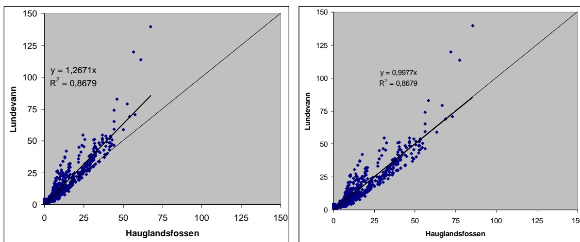
Figur 5. Vannføring målt ved Hauglandsfossen og ved NVEs stasjon 18.4.0. I figuren til venstre (a) er ukorrigert data fra Hauglandsfossen vist. I figuren til høyre (b) er vannføringen økt med en faktor på 1,27.
