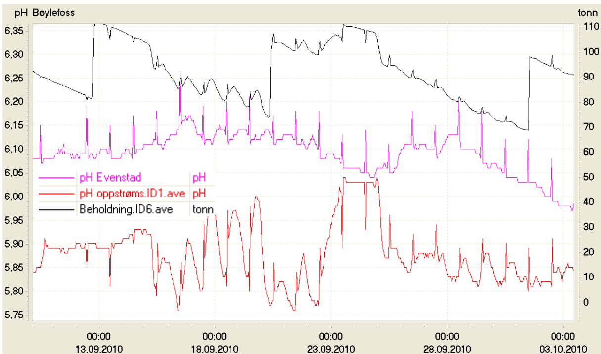
Figur 2. Signalforstyrrelser resulterte i feil på tre parametere: pH-Evenstad, pH oppstrøms anlegget og kalkbeholdning. Årsaken til forholdet er ikke kjent.
