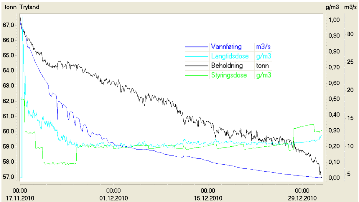
Figur 5. Vannføring, beholdning, styringsdose og langtidsdose fra tidspunktet da doseringssignalet ble etablert som parameter i driftskontrollen.
