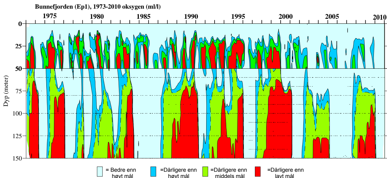
Figur 33. Oksygenkonsentrasjonen i Bunnefjorden (Ep 1) 1973-2010 sammenlignet med miljømålene (Bjerkeng mfl., 2009). Det er høyere krav til oksygen fra 20-50 meters dyp enn fra 50-150 meters dyp. Figuren viser at oksygenkonsentrasjonen dypere enn ca. 60 m varierer mye fra år til år. I 2010 oppfylte dypvannet høyt mål. Imidlertid synes vannmassen mellom 20-60/70 meters dyp å oppfylle kravet til lavt mål siden 2004, med flere år som tilfredsstillte middels mål. For dypvannet er dårligere enn lavt mål lik med forekomsten av hydrogensulfid.
