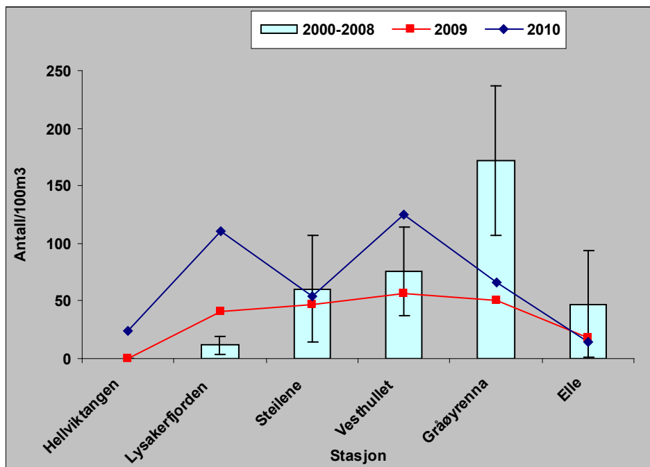
Figur 73. Gjennomsnittlig antall arter av reker pr sledetrekk (øverst) og gjennomsnittlig antall individer pr 100 m 3 "filtrert" vann for innsamling med slede foretatt i perioden 2000-2008. Konfidensintervall (95 %) er inntegnet. Verdiene for 2009 og 2010 er vist separat.
