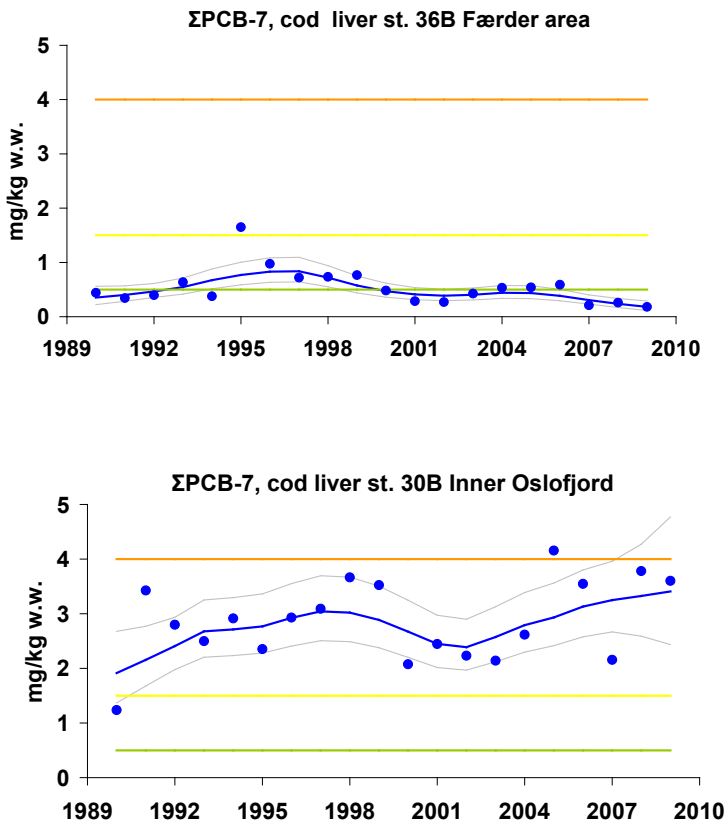
Figur 5. Konsentrasjonen av sum PCB-7 i torskelever fra Færder (øverst) og Indre Oslofjord (nederst) fra 1990 til 2009. Grenser for grad av forurensning er markert (verdier under grønn linje: ubetydelig til lite forurensset, verdier mellom grønn og gul linje: moderat forurensset, verdier mellom gul og orange linje: markert forurensset, verdier over orange linje: sterkt forurensset). Data fra NIVA/Klif, rapport TA-2716/2010.
