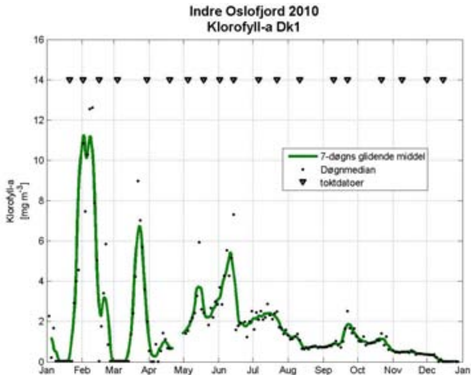
Figur 54. Døgnsmedian og 7 døgns glidende middel av klorofyll-a ( \mu\text{g/l} ) i ca. 4 meters dyp i Vestfjorden (Dk1) observert med FerryBox i 2010. Observasjonene er omregnet fra klorofyll-a fluorescensmålinger til klorofyll-a etter kontrollprøvetaking (analyser av klorofyll-a fra vanninntak om bord i Color Fantasy). Tidspunkt for ferryboxtoktene er markert.
