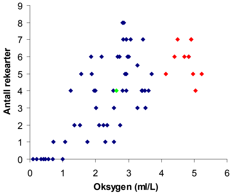
Figur 83. Totale antall rekearter per sledetrek (ca 1000 m) på stasjoner fra Bunnefjorden (Hellviktangen) til Drøbaksundet (Elle) i perioden 2000-2010 som funksjon av oksygenkonsentrasjonen i vannet rett over bunnen. Data fra Elle i Drøbaksundet er merket med rødt og grønt (2010 data)
