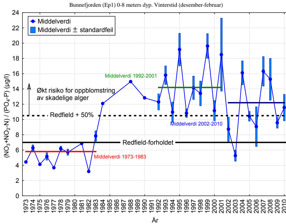
Figur 67. Vinterobservasjoner av \text{NO}_3+\text{NO}_2\text{-N}/\text{PO}_4\text{-P} (DIN/DIP) i Bunnefjorden (Ep 1) i 0, 4 og 8 meters dyp 1973-2010. N/P-forholdet øker signifikant i perioden og ligger i 1992-2001 ofte mer enn 50 % over Redfieldforholdet. Etter OSPAR (2001) vil et DIN/DIP-forhold større enn Redfieldforholdet + 50 % øke risikoen for oppblomstring av skadelige alger. Etter 2001 er det store variasjoner med tendens til noe lavere N/P-forhold.
