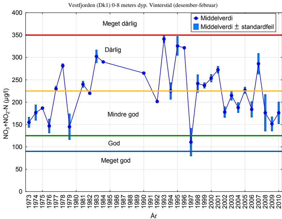
Figur 63. Vinterobservasjoner av \text{NO}_3+\text{NO}_2\text{-N} i Vestfjorden (Dk 1) i 0, 4 og 8 meters dyp 1973-2010. Utviklingen er sammenlignet med Klifs miljøklassifiseringssystem for vannkvalitet. Vannkvaliteten varierer fra dårlig til mindre god , og det er ingen endring fra 1970-tallet til perioden 2002-2009, men
