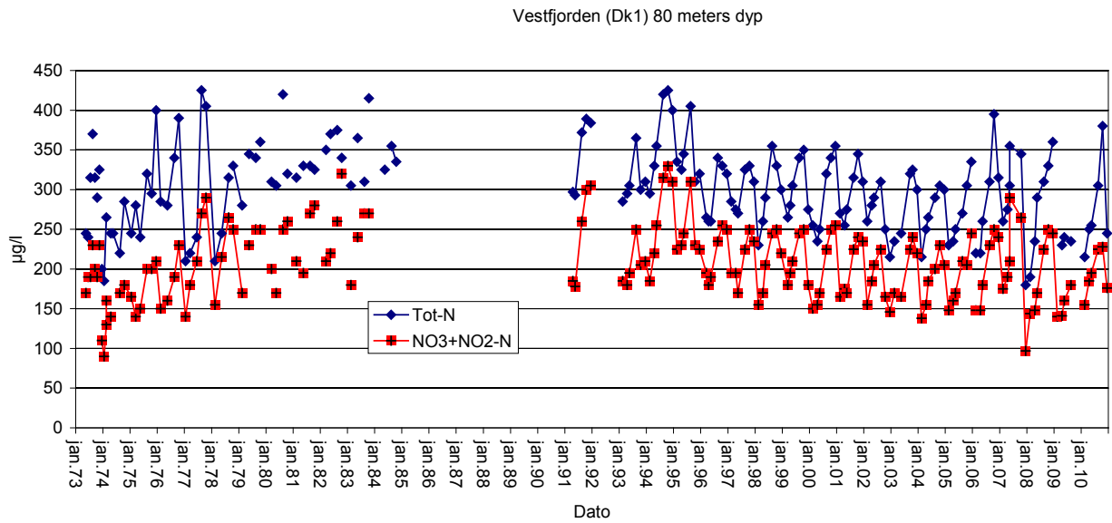
Figur 52. Tot-N og \text{NO}_3+\text{NO}_2\text{-N} ( \mu\text{g/l} ) på 80 meters dyp i 1973-2010.
