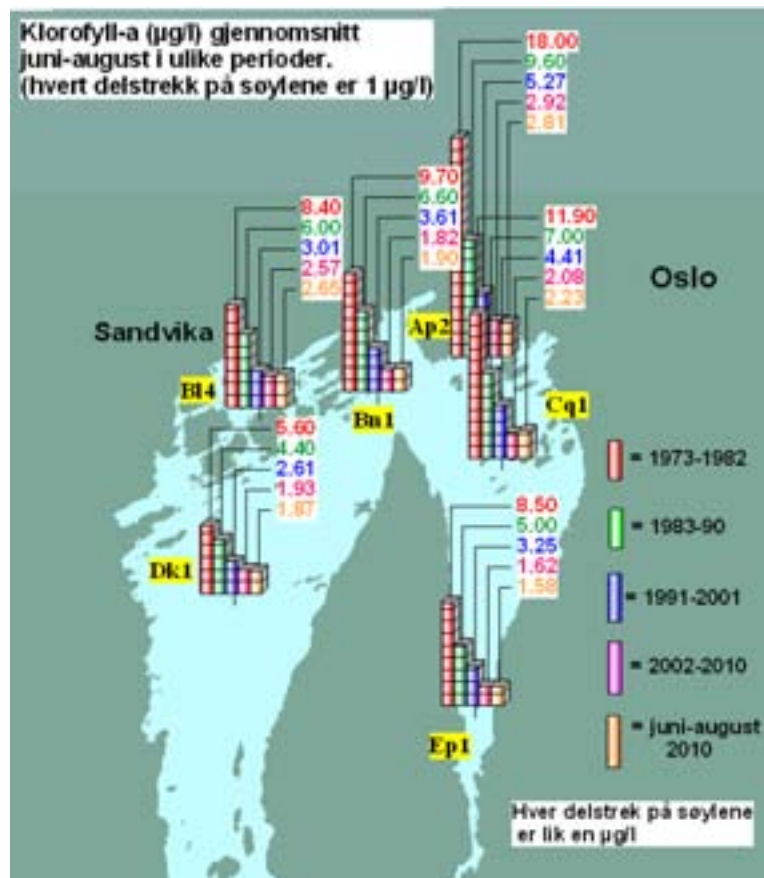
Figur 58. Klorofyll-a ( \mu\text{g/l} ) i 0-2 meters dyp, middelverdier i juni-august fra 1973-82, 1983-90, 1991-2001, 2002-2010 og 2010. Klorofyll-a er et indirekte mål på planteplanktonbiomassen.
