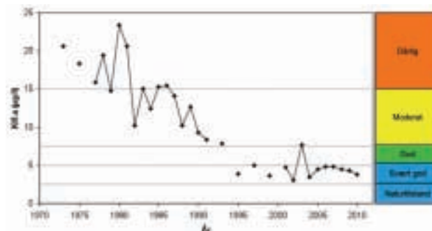
Figur 4. Konsentrasjon av klorofyll-a i Gjersjøen for perioden 1972-2010 (middelverdier 0-10 meters dyp), samt grensene mellom de ulike økologiske tilstandsklassene i klassifiseringssystemet til Vanndirektivet.
