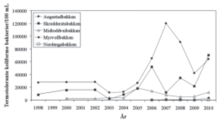
Figur 7. 90-percentiler for innhold av tarmbakterier i Kolbotnbekken i perioden 1998-2010.
