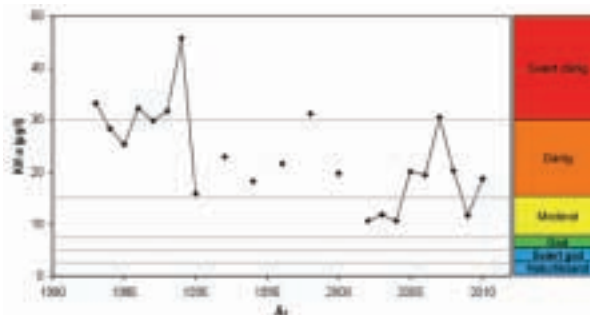
Figur 13. Konsentrasjon av klorofyll-a i Kolbotnvannet for perioden 1972-2010 (middelverdier 0-4 meters dyp), samt grensene mellom de ulike økologiske tilstandsklassene i klassifiseringssystemet til Vanndirektivet (referansetilstanden, svært god (SG), god (G), moderat (M), dårlig (D)).
