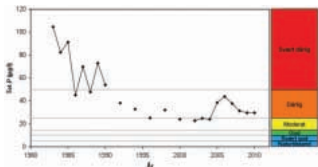
Figur 12. Målte konsentrasjoner av total fosfor (µg/L) i Kolbotnvannet (0-4 meter) for perioden 1984-2010, samt grensene mellom de ulike økologiske tilstandsklassene i klassifiseringssystemet til Vanndirektivet.
