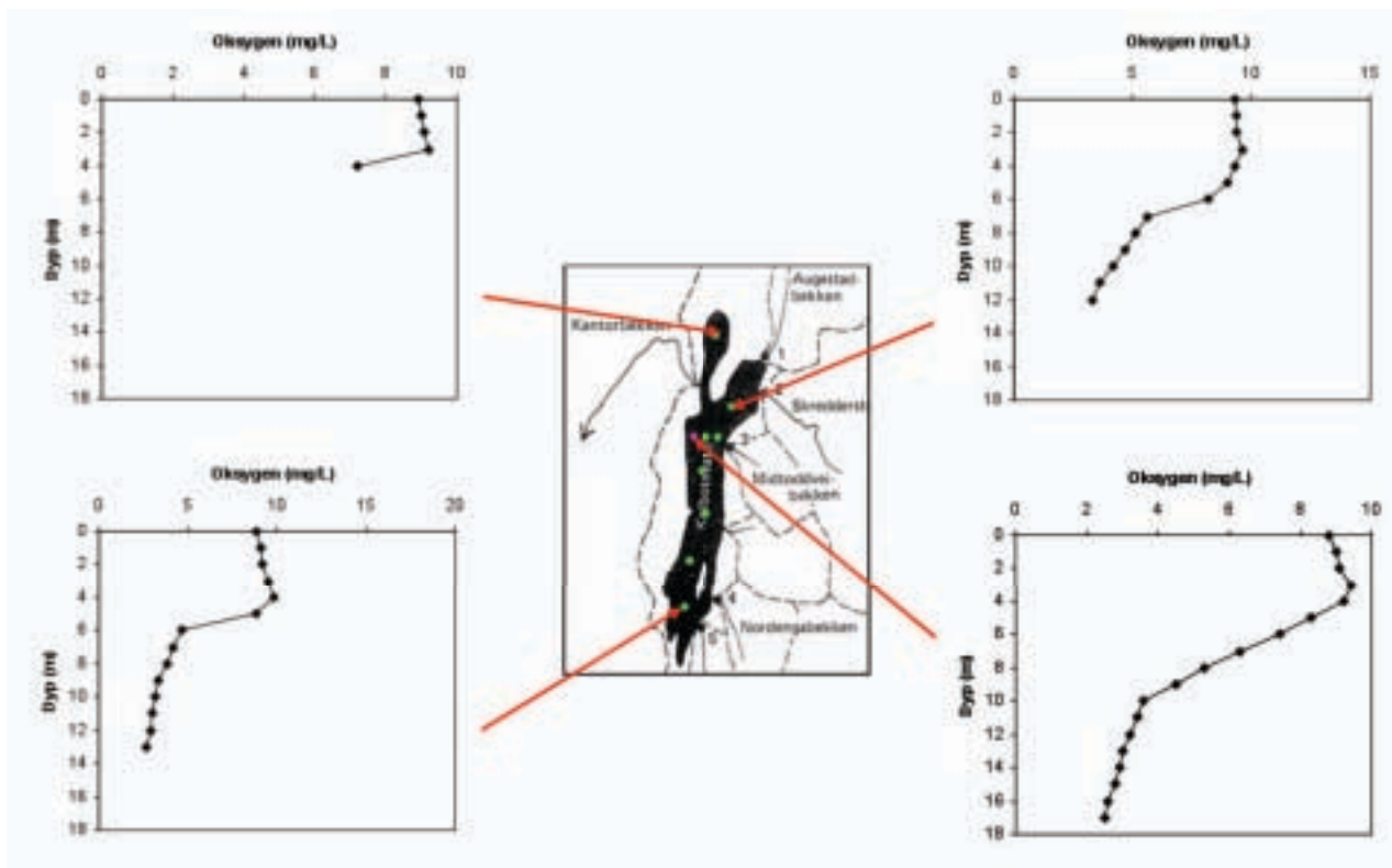
Figur 9. Oksygenprofiler på flere stasjoner i Kolbotnvannet den 30.06.2010
