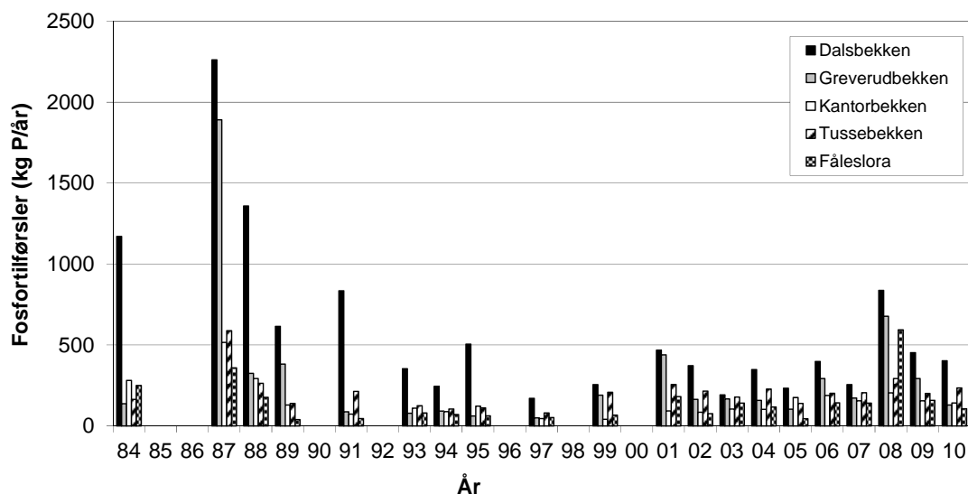
Figur 5. Fosfortilførsler til Gjersjøen fra hver av tilløpsbekkene i perioden 1984-2010.
