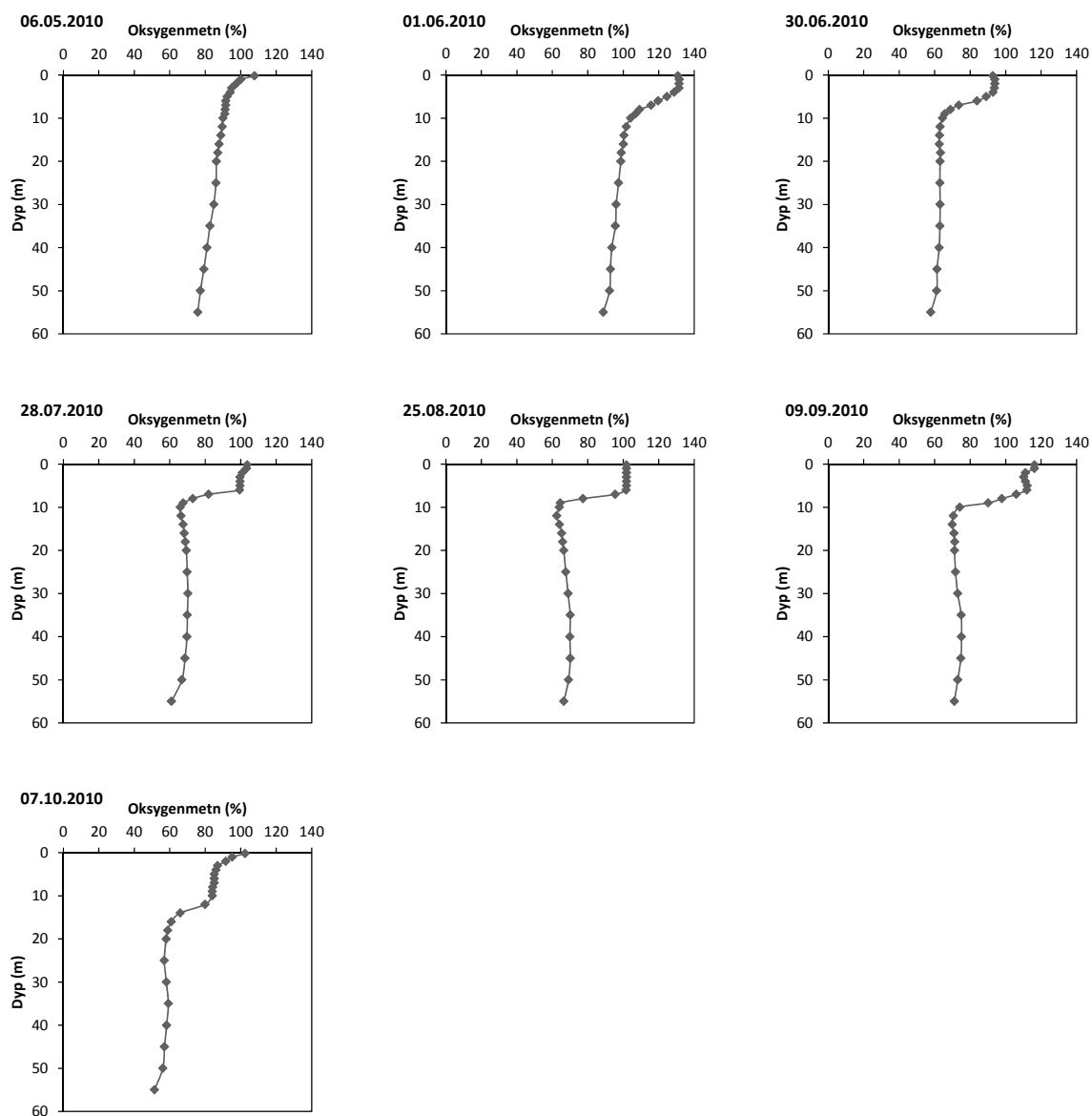
Figur 8. Oksygenvertikalsnitt for Gjersjøen i 2010.
