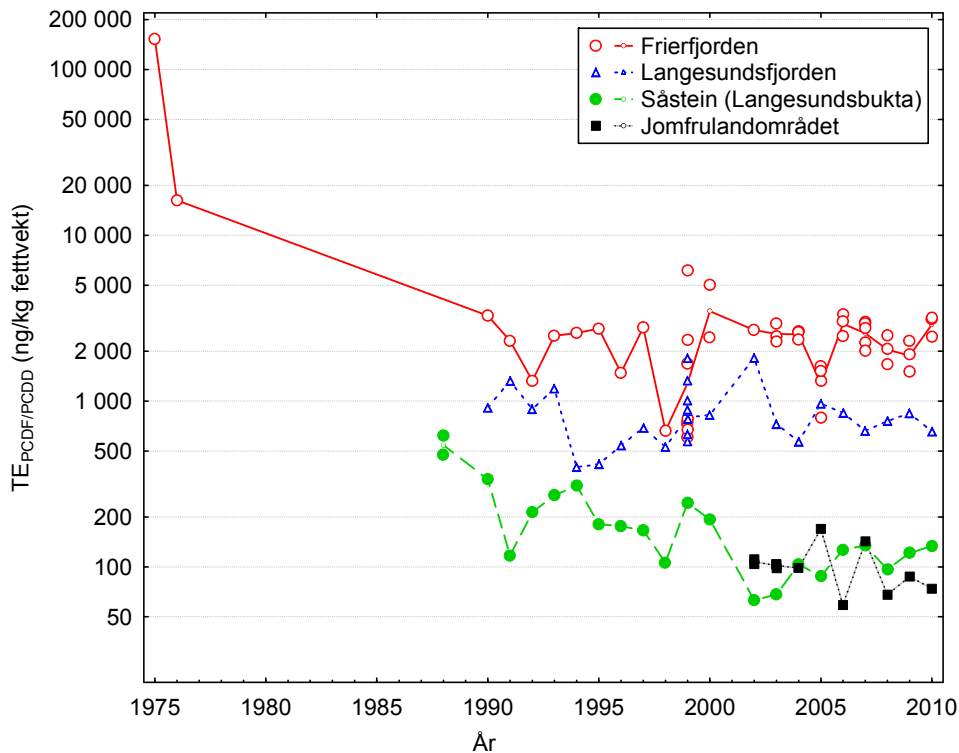
Figur 4. Dioksiner i torskelever på fettvektbasis (ngTE/kg fettvekt) som funksjon av tid til og med 2010. Alle replikater er vist (men ikke "fettrik" og "fettfattig" prøve); linjene er trukket mellom gjennomsnittsverdier på log-skala, dvs. geometrisk middel på lineær skala. NB: den logaritmiske skalaen på y-aksen demper inntrykket av reduksjonen over tid.
