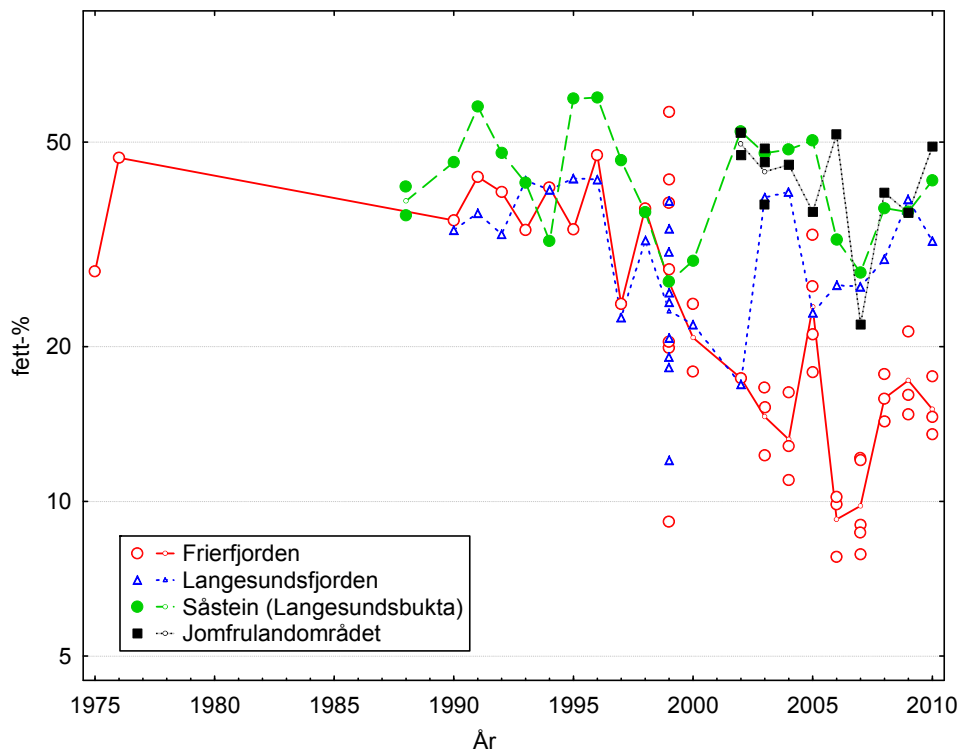
Figur 3. Fettinnhold i torskelever (%) som funksjon av tid til og med 2010. Alle replikater er vist (men ikke "fettrik" og "fettfattig" prøve); linjene er trukket mellom gjennomsnittsverdier.
