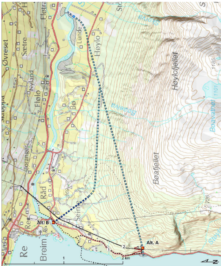
Figur 3. Omsøkt plassering av inntak og kraftstasjon med utløp i Breimsvatnet (A). Alternativ plassering av kraftstasjon med utløp ved Seime bru (B) er utredet, men ikke omsøkt. Figur utarbeidet av Multiconsult.
