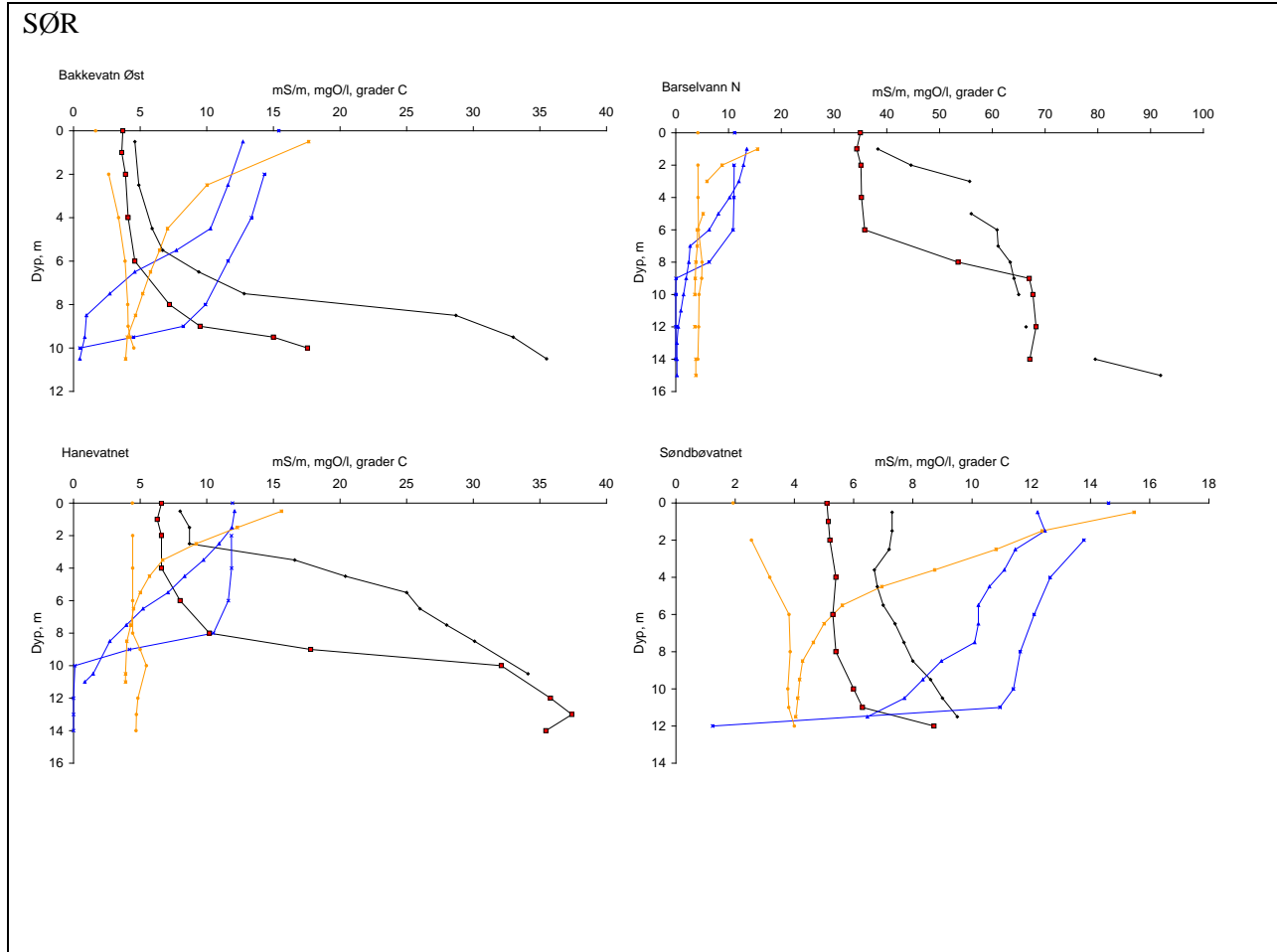
Figur 12. Dybdeprofiler av konduktivitets, oksygen og temperatur for vår/tidlig sommer og sen høst for 4 Innsjøer fra hver region. Merk at skalaene er forskjellige.
