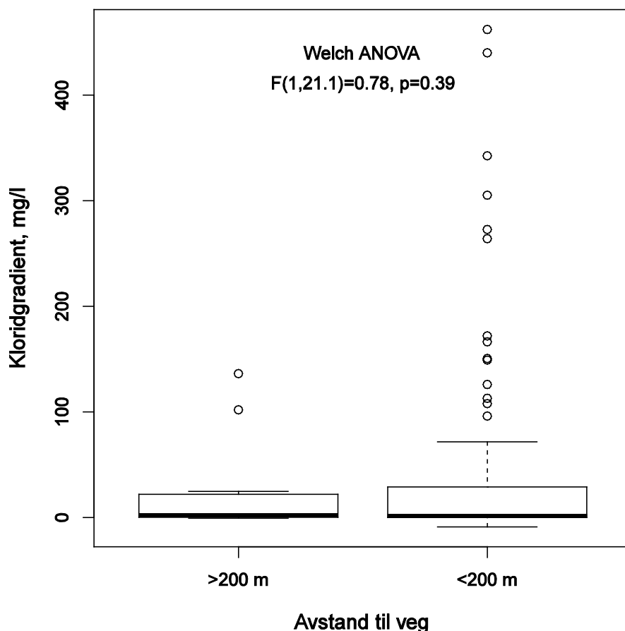
Figur 15. Box plott av kloridgradienter ( [Cl]_{\text{bunn}} - [Cl]_{\text{overflate}} ) for innsjøer som ligger mer enn 200 meter unna veg ( n=12 ) og innsjøer som ligger mindre enn 200 meter unna veg ( n=82 ). Tilhørende teststatistikk for Welch ANOVA som tester forskjell mellom de to innsjøkategoriene er oppgitt. Welch ANOVA tillater ulik innen-gruppe varians for de to gruppene.
