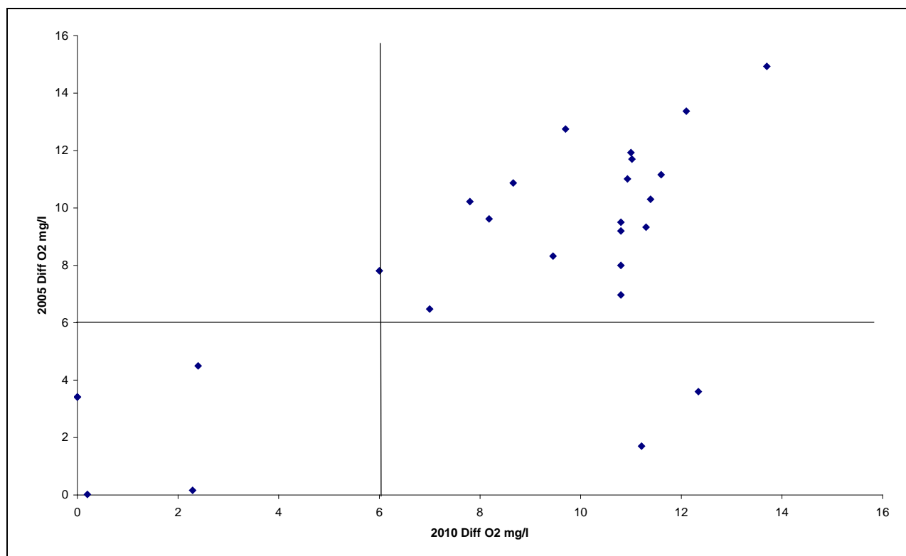
Figur 9. Oksygengradient (overflatevann – bunnvann) i 26 innsjøer undersøkt både i 2005 og 2010. Linjer viser oksygengradient på 6 mg O/l.
