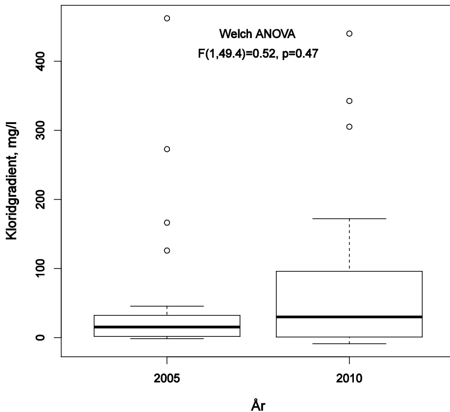
Figur 14. Box plott av kloridgradienter ( [Cl]_{\text{bunn}} - [Cl]_{\text{overflate}} ) for innsjøer ( n=26 ) som ble målt i både 2005 og 2010 samt teststatistikk for Welch ANOVA som tester forskjell mellom de to åra. Welch ANOVA tillater ulik innen-gruppe varians for de to gruppene.
