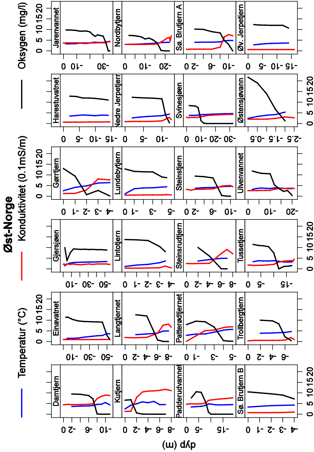
Figur 2 A-C. Regionvis profilplott av konduktivitet, temperatur og oksygen for alle innsjøer som ble målt i 2010.
