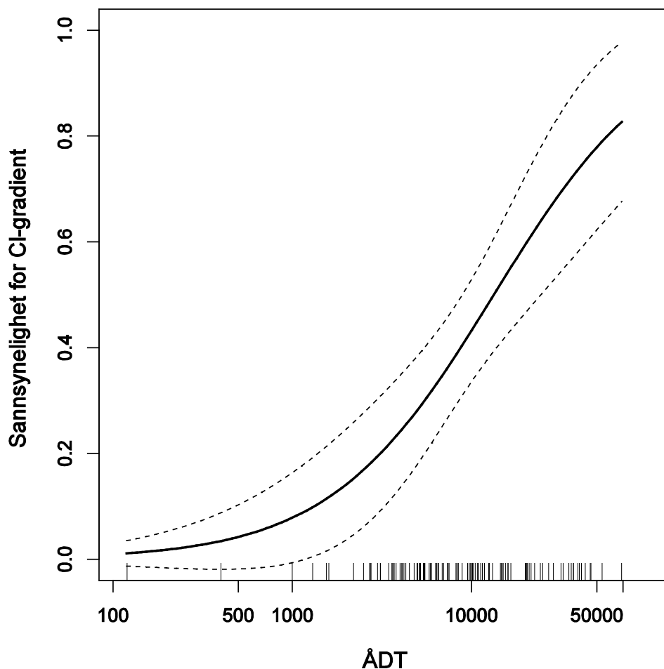
Figur 17. Estimert sannsynlighet for at en innsjø skal ha kloridgradient som funksjon av trafikkmengde (ÅDT) på innsjøens nærmeste veg. Estimateret er avledet ved logistisk regresjon der en innsjø sies å ha kloridgradient dersom [Cl]_{\text{bunn}} - [Cl]_{\text{overflate}} > 10 \text{ mg/l} (Bækken og Haugen 2006). ÅDT forklarer 12 % av variasjonen.
