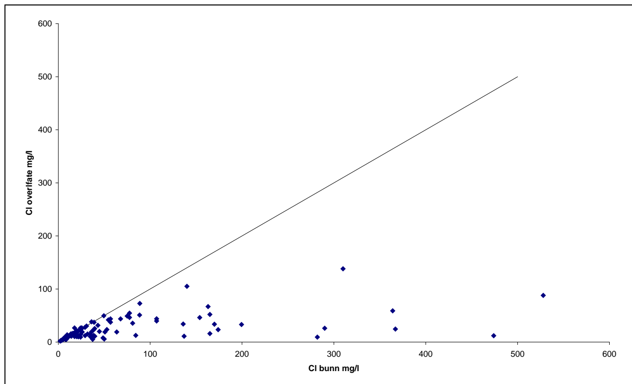
Figur 3. Fordelingen av klorid i overflatevannet og bunnvannet i 121 innsjøer. 26 av disse er prøvetatt både i 2005 og 2010. Linje angir forholdet 1:1.
