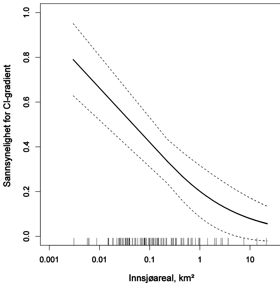
Figur 16. Estimert sannsynlighet for at en innsjø skal ha kloridgradient som funksjon av innsjøens areal. Estimaten er avledet ved logistisk regresjon (GLM, logit) der en innsjø sies å ha kloridgradient dersom [Cl]_{\text{bunn}} - [Cl]_{\text{overflate}} > 10 mg/l (Bækken og Haugen 2006). Stiplede linjer angir 95 % - konfidensintervall. Modellen forklarer 9 % av variasjonen.
