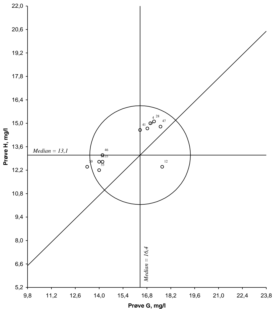
Figur 26. Youdendiagram for kjemisk oksygenforbruk, \text{COD}_{\text{Mn}} , prøvepar GH Akseptansegrensen, angitt med en sirkel, er 20 %
