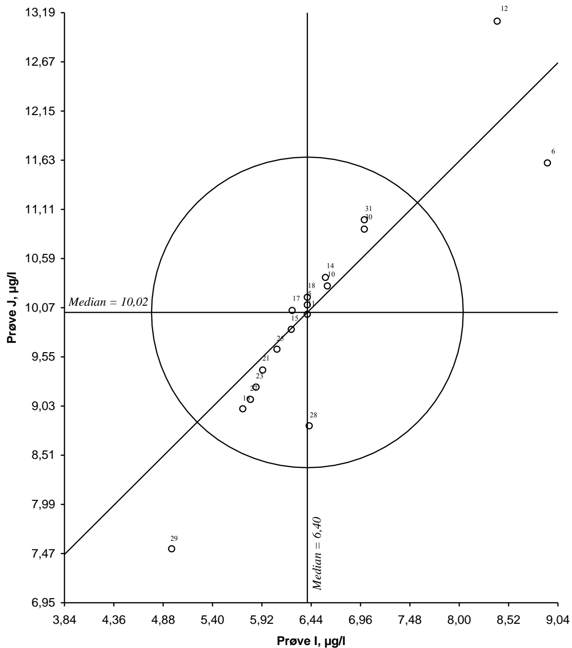
Figur 39. Youdendiagram for bly, prøvepar IJ Akseptansegrensen, angitt med en sirkel, er 20 %
