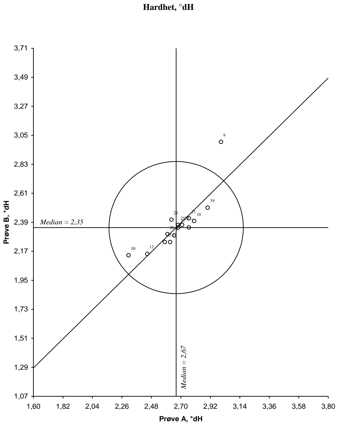
Figur 13. Youdendiagram for hardhet, °dH, prøvepar AB Akseptansegrensen, angitt med en sirkel, er 20 %
