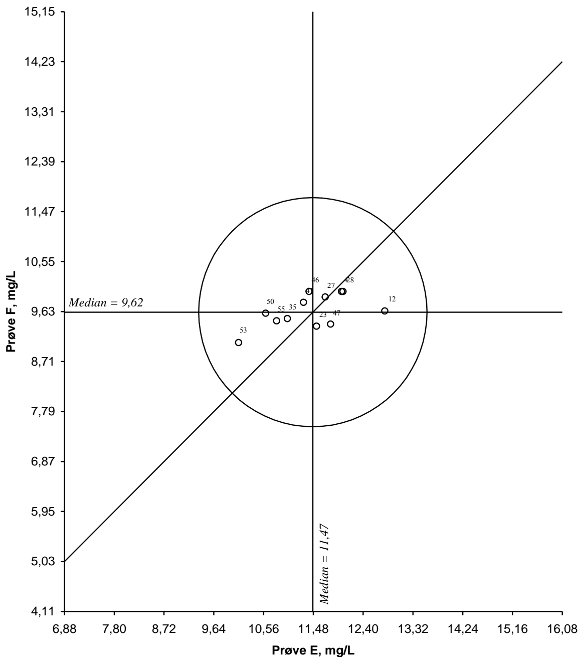
Figur 25. Youdendiagram for kjemisk oksygenforbruk, COD Mn , prøvepar EF Akseptansegrensen, angitt med en sirkel, er 20 %
