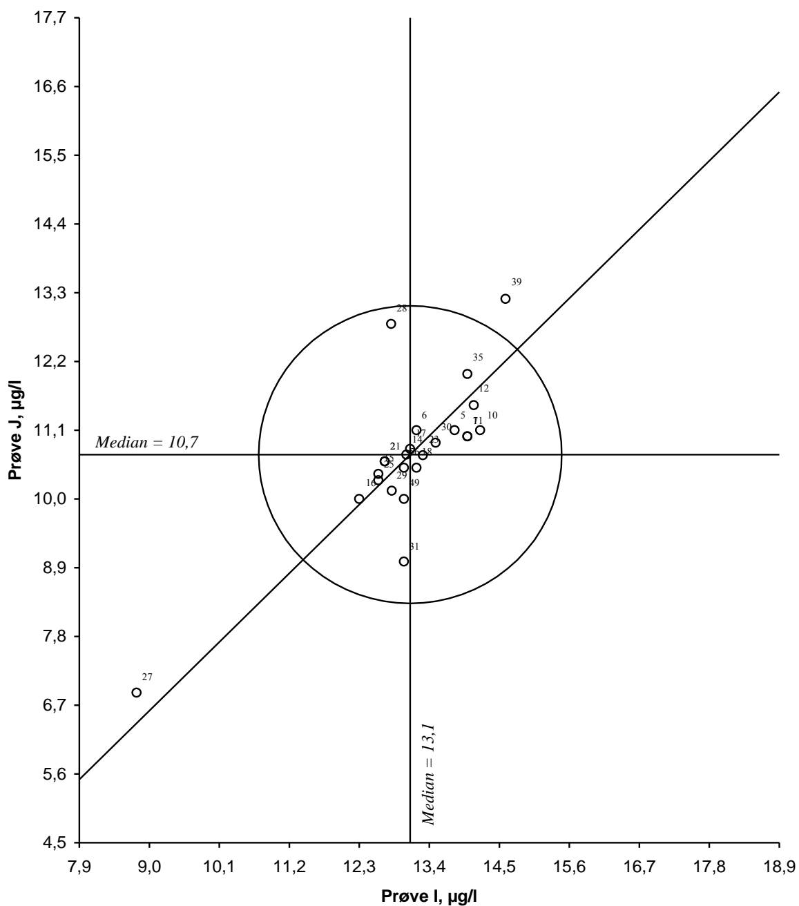
Figur 49. Youdendiagram for mangan, prøvepar IJ Akseptansegrensen, angitt med en sirkel, er 20 %
