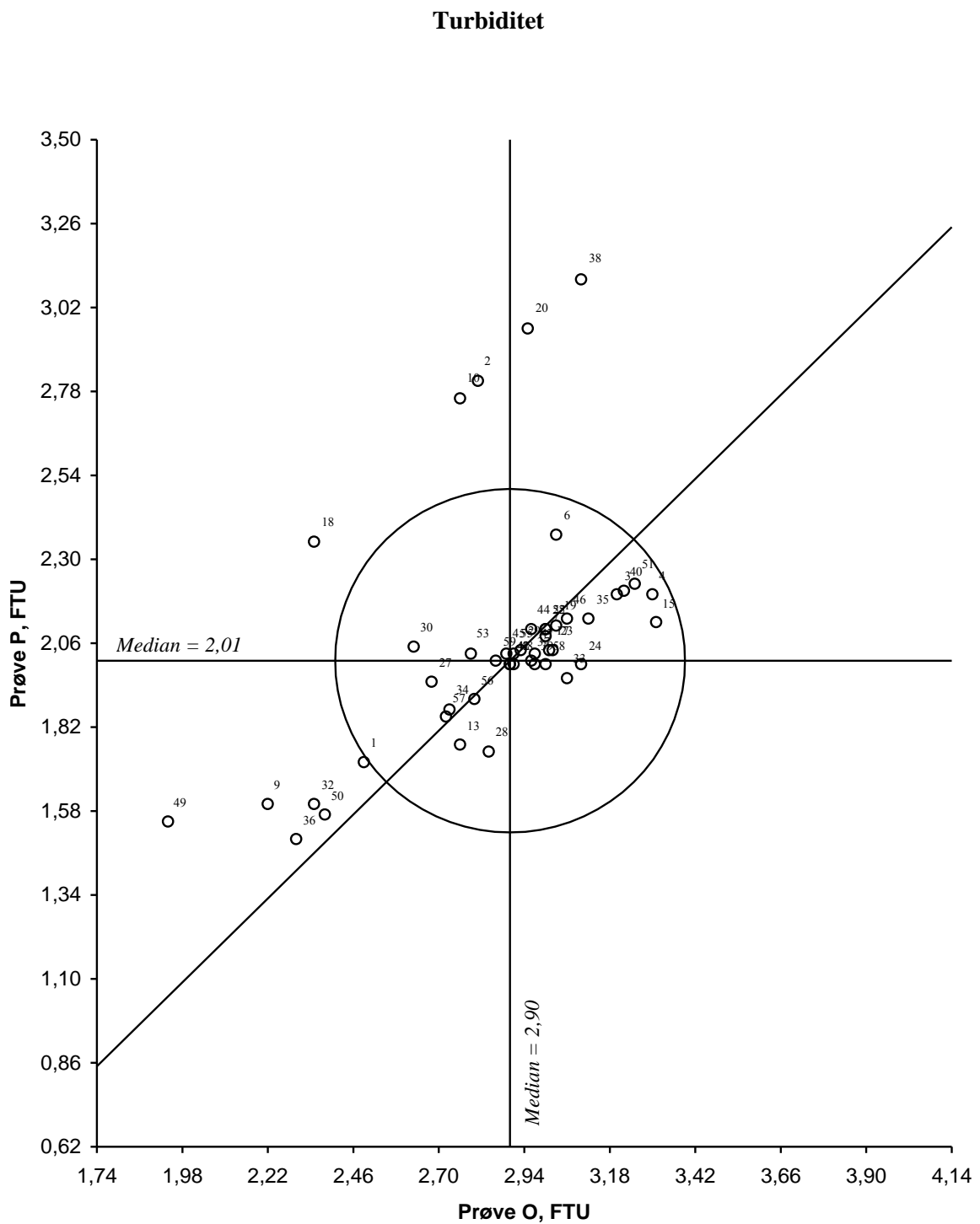
Figur 59. Youdendiagram for turbiditet, prøvepar OP Akseptansegrensen, angitt med en sirkel, er 20 %
