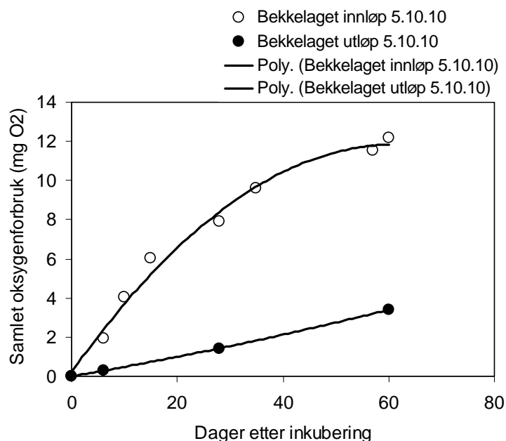
Figur 8. Typisk forløp for oksygenforbruket under lab-forsøkene ved bestemmelse av totalt oksygenforbruk på grunn av organisk karbon ( TOF_{OC,spe} ).
