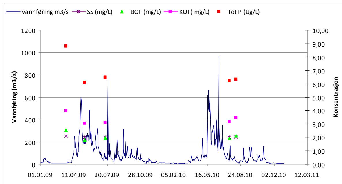
Figur 4. Vannføringen i Gaula ved Gaulfoss i undersøkelsesperioden med innlagte konsentrasjoner for tot-P, KOF, BOF og SS etter innblanding av utslippene fra Norsk Kylling AS og Moøya renseanlegg.
