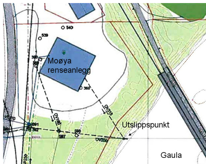
Figur 3. Utslippspunkt Møya rensanlegg.
