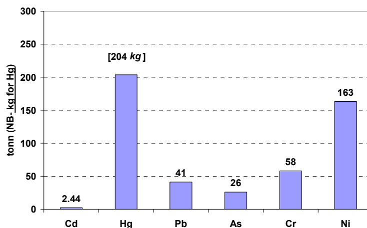
Figur 9. Totale årlige tilførsler av kadmium (Cd), kvikksølv (Hg), bly (Pb), arsen (As), krom (Cr) og nikkel (Ni) til havområdene i perioden 2005-2009 (nedre estimater). Merk at verdien for kvikksølv er gitt i kilo, øvrige verdier i tonn.
