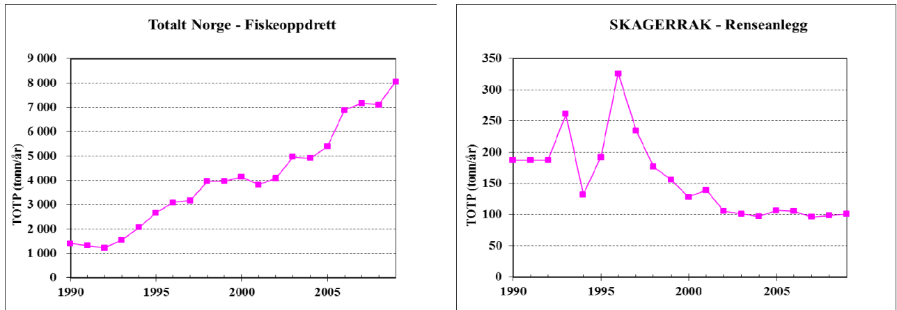
Figur 16. Tilførsler av totalfosfor for hele Norge fra fiskeoppdrett (venstre) og til Skagerrak fra renseanlegg (høyre), 1990-2009.
