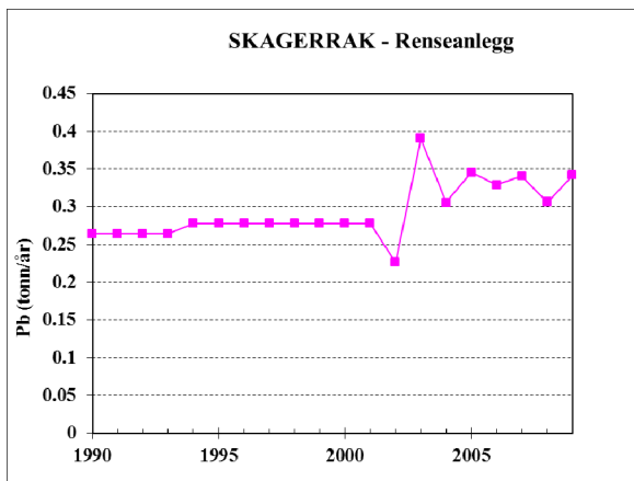
Figur 25: Tilførsel av bly fra renseanlegg (venstre) og industri (høyre) til Skagerrak
