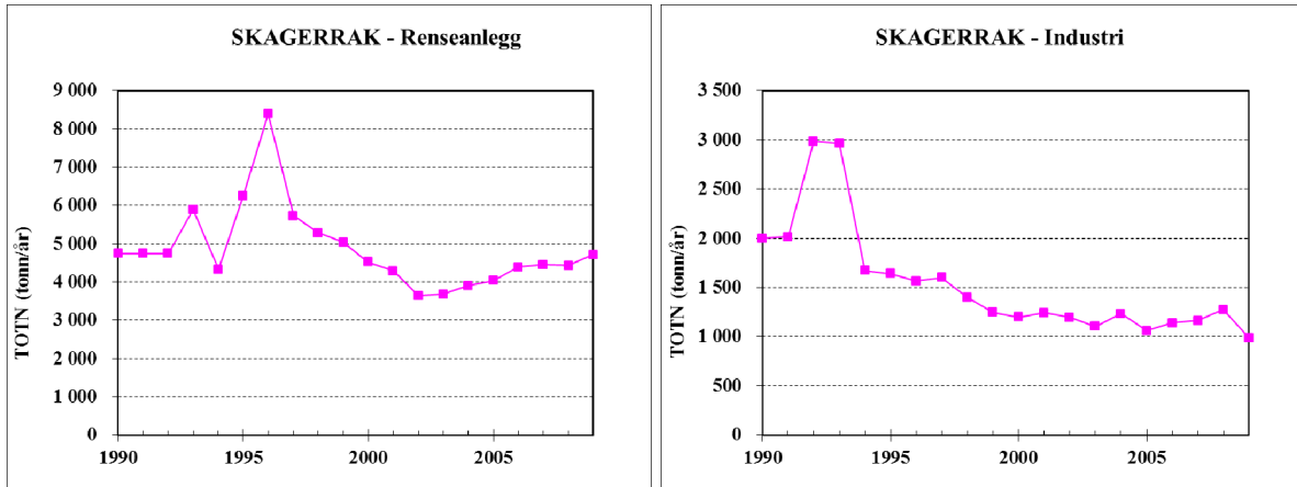
Figur 13: Tilførsler av total nitrogen fra renseanlegg og industri til Skagerrak 1990-2009.
