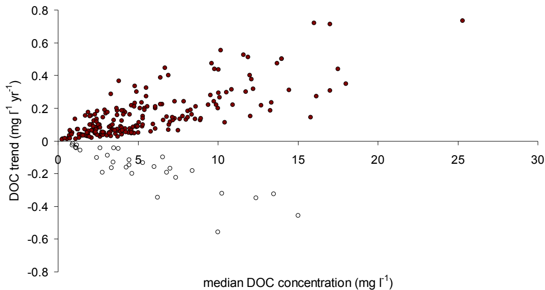
Figur 2. Forhold mellom løst organisk karbon (DOC) trender ( \text{mg C/L/år} ) og absolutt DOC-konsentrasjon (median verdi for hver lokalitet over perioden 1990-2004). Positive og negative trender ( p < 0,1 ) er angitt ved henholdsvis hele og åpne sirkler. Kilde: (Monteith et al. 2007) i ICP Waters report 87/2007 (de Wit and Skjelkvåle 2007).
