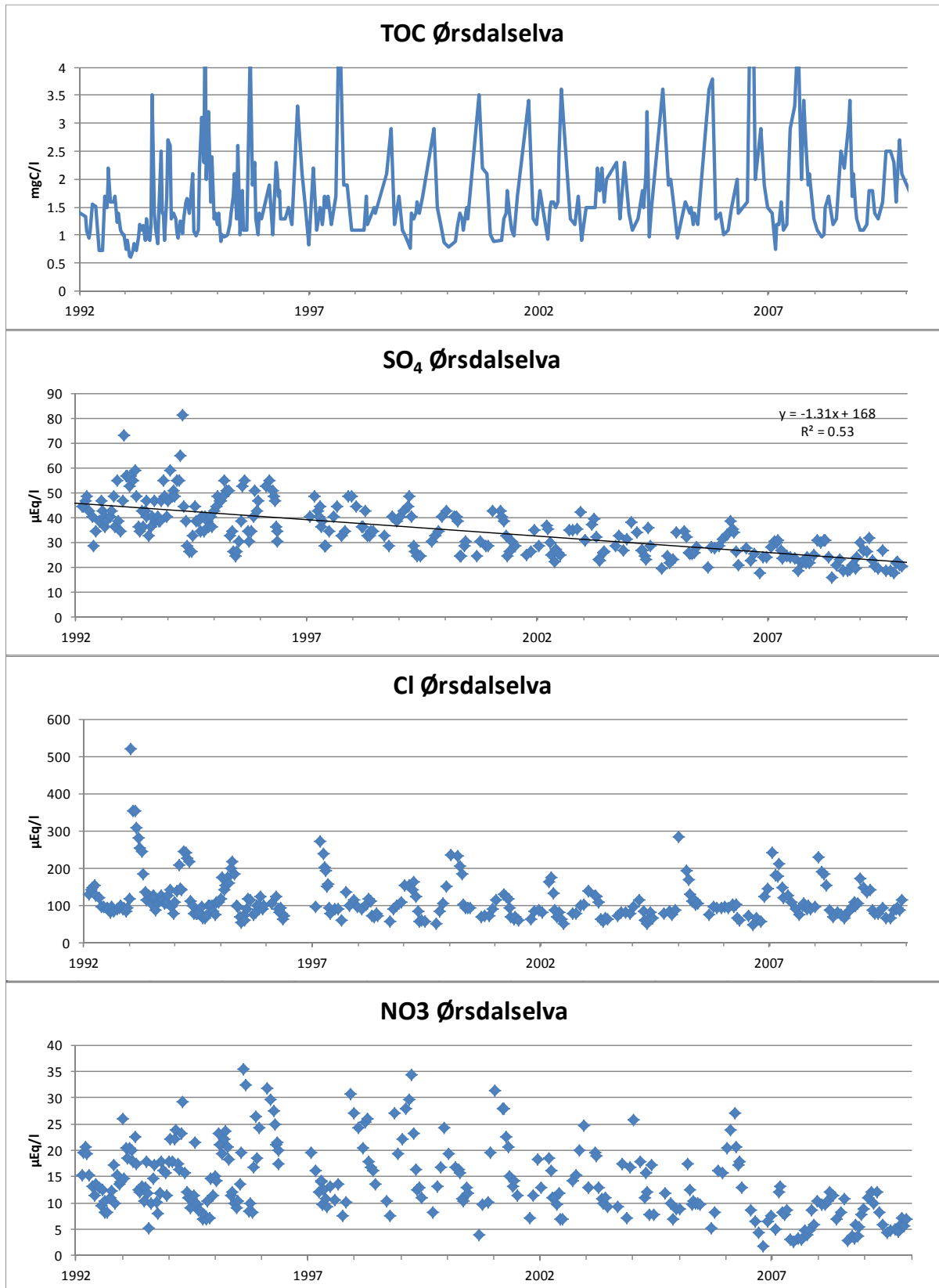
Figur 9. Konsentrasjoner av TOC, SO 4 , Cl, og NO 3 i Ørsdalselva for perioden 1992-2010.
