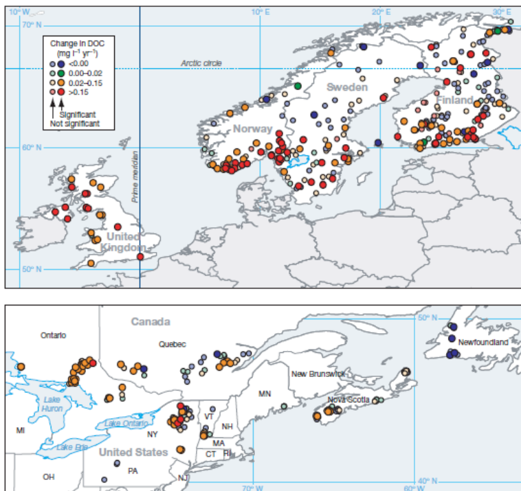
Figur 1. Trender i løst organisk karbon (DOC) ( \text{mg/l/år} ) i innsjøer i nord Europa og østlige Nord-Amerika i perioden 1990-2004. Kilde: Monteith et al. (2007)
