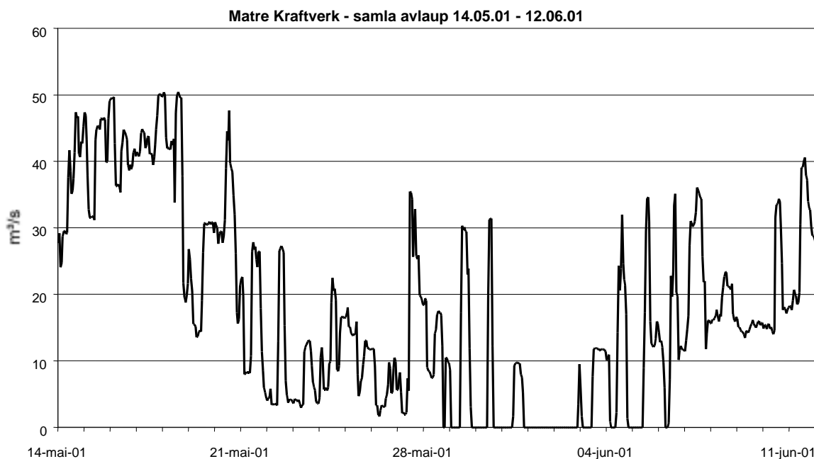
Figur 7. Døme på variasjon i avlaup fra Matre Kraftverk (mai-juni 2001, \text{m}^3/\text{s} ). Merk periodane med stans i kraftproduksjonen. Data fra BKK.
