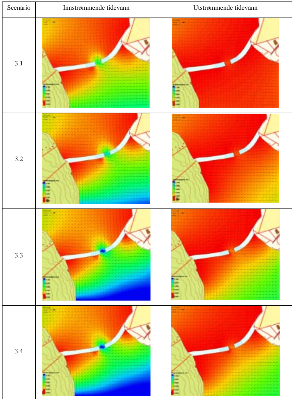
Figur 21. Scenario 3: Gjennomstrømming i 20 m bred åpning i fyllinga mellom fastlandet og Matresøyna. Figurene beskriver 4 kombinasjoner av vannføring i elva og utslipp fra kraftverket (S3.1-3.4, jfr. Tabell 4). For hver kombinasjon vises to figurer, med innstrømmende tidevann til venstre og utstrømmende tidevann til høyre. Merk at fargeskalaen her er annerledes enn i foregående figur.
