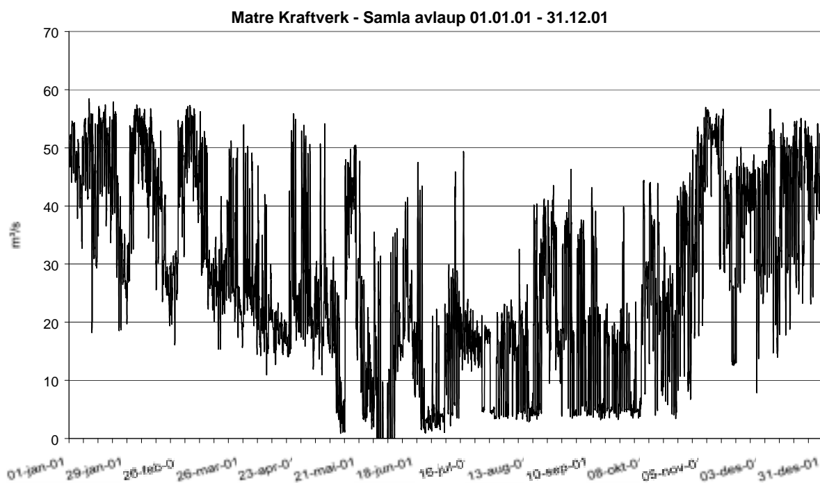
Figur 6. Avlaup ( \text{m}^3/\text{s} ) fra Matre Kraftverk i år 2001. Data fra BKK.
