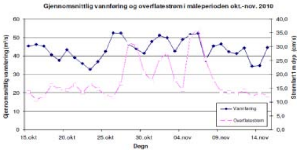
Figur 16. Gjennomsnittlig vannføring ( m^3/s/døgn ) fra kraftverket i Matre og gjennomsnittlig strømhastighet ( cm/s/døgn ) på 1 meters dyp ved Matresøyna sør i perioden 14. oktober – 15. november 2010.
