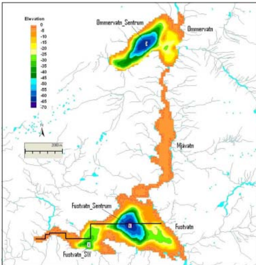
Figur 10. Lengde-dybdessnitt og profiler. Stedsangivelse for resultater vist i under.
