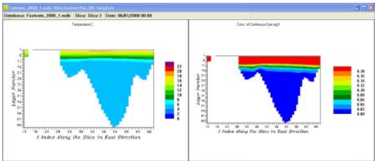
Figur 6. Dybdesnitt vest – øst over dypeste del av innsjøen. Temperatur og konsentrasjon av et kontinuerlig dosert konservativt stoff i de største tilløpselvene 1. mai 2008. Overflatevannet ble varmet opp, ble lettere slik at ellevannet la seg nær overflaten.
