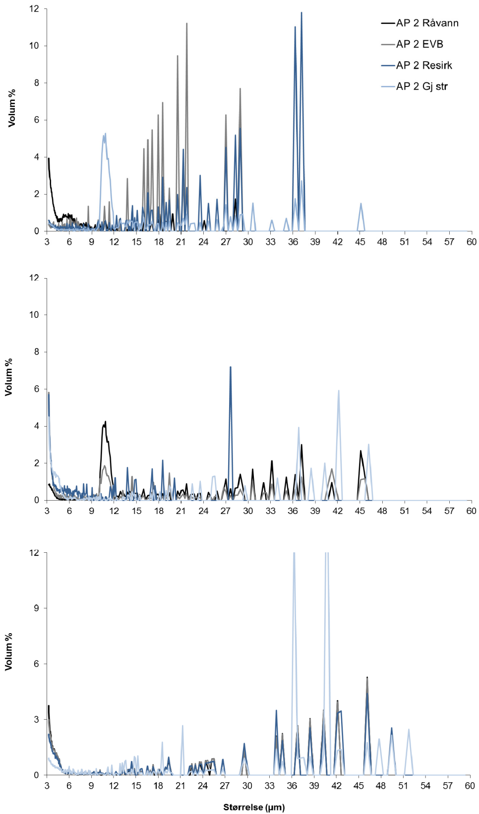
Figur 10. Volumfordeling (%) av partikler (3,2-60 \mu\text{m} ) i Råvann, Etter vannbehandling, Resirkulasjonssystemet og Gjennomstrømmingssystemet ved start, etter 3 uker og slutt i forsøk 2.
