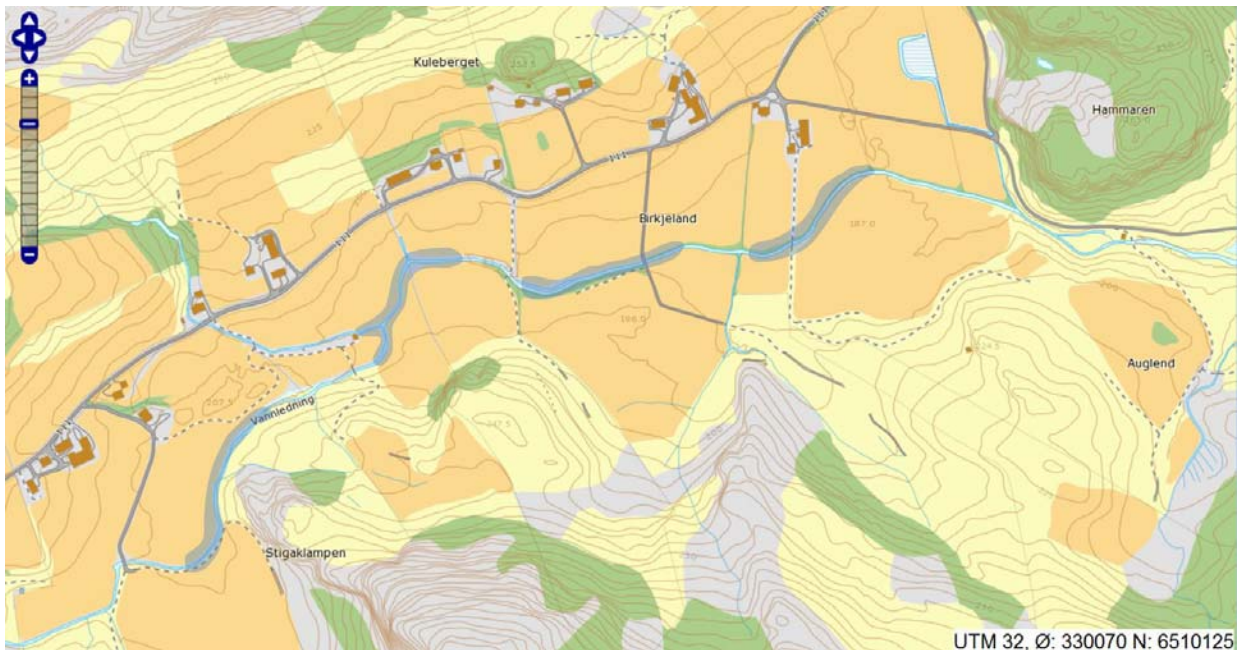
Figur 27. Nedrebøelva med angivelse av mulige konstruerte fangdammer, forutsatt at vannet fra kraftverksutløpet ledes til Storavatnet i rør. NB - det må gjøres en befaring i felt for å anslå plasseringene mer nøyte. Her er det kun gjort vurderinger ut fra kart.
