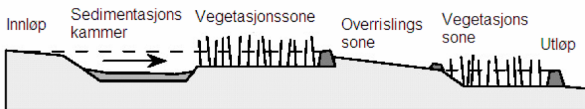
Figur 26. Oppbygning av en fangdam etter Bioforsk Tema 3 (13), 2008.
