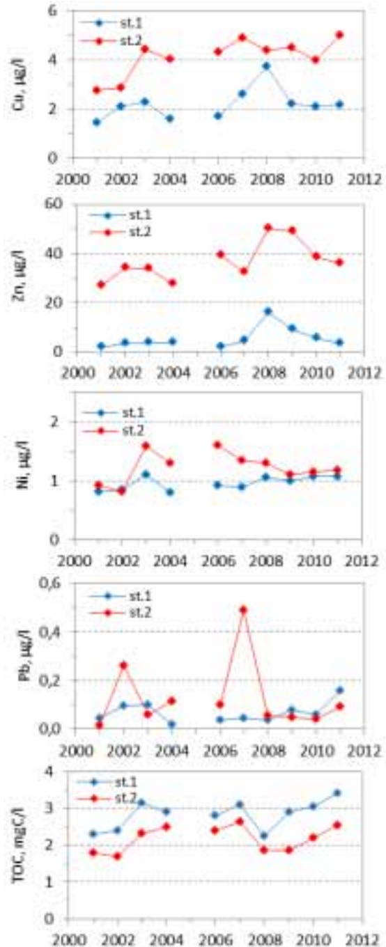
Figur 7. Middelkonsentrasjoner (mai-okt.) av kobber (Cu), sink (Zn), nikkel (Ni), bly (Pb) og totalt organisk karbon (TOC) i bekken oppstrøms (blå kurver) og nedstrøms (rød kurver) Grisungdalen demoleringsfelt i Hjerkinnskytefeltet i perioden 2001-2011.
