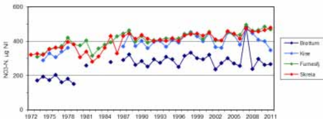
Figur 14. Tidsutviklingen i middelverdier for nitrat fra målinger på senvinteren i perioden 1971-2011 (basert på målinger fra overflate til nær bunn).
