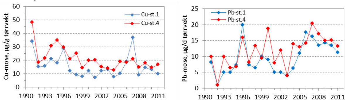
Figur 3. Middelskonsentrasjonene av kobber (Cu) og bly (Pb) i vannmoser ved stasjon 1 (inn i feltet) og 4 (ut av feltet) i Veltmannåa. Fra og med 2006 er konsentrasjonene estimert (se metodekapitlet).
