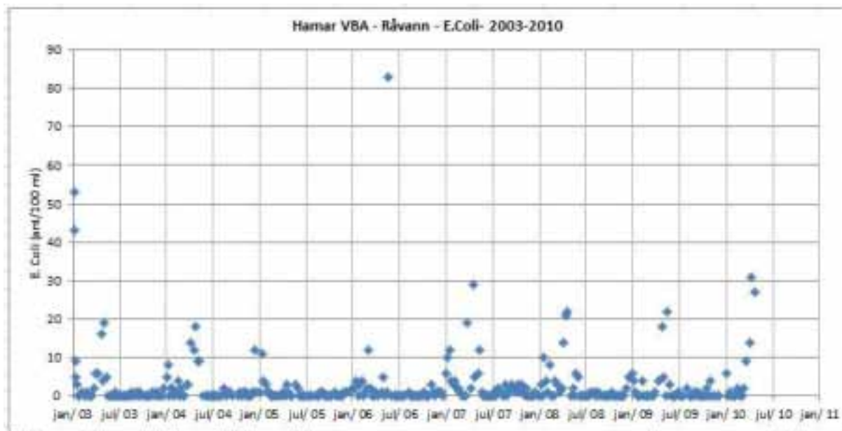
Figur 13. Observerte E. coli verdier i råvannsinntaket til Hamar vannverk 2003 – 2011. Vanninntaket ble sporadisk påvirket. Det var mest utsatt under vårsirkulasjonen.
