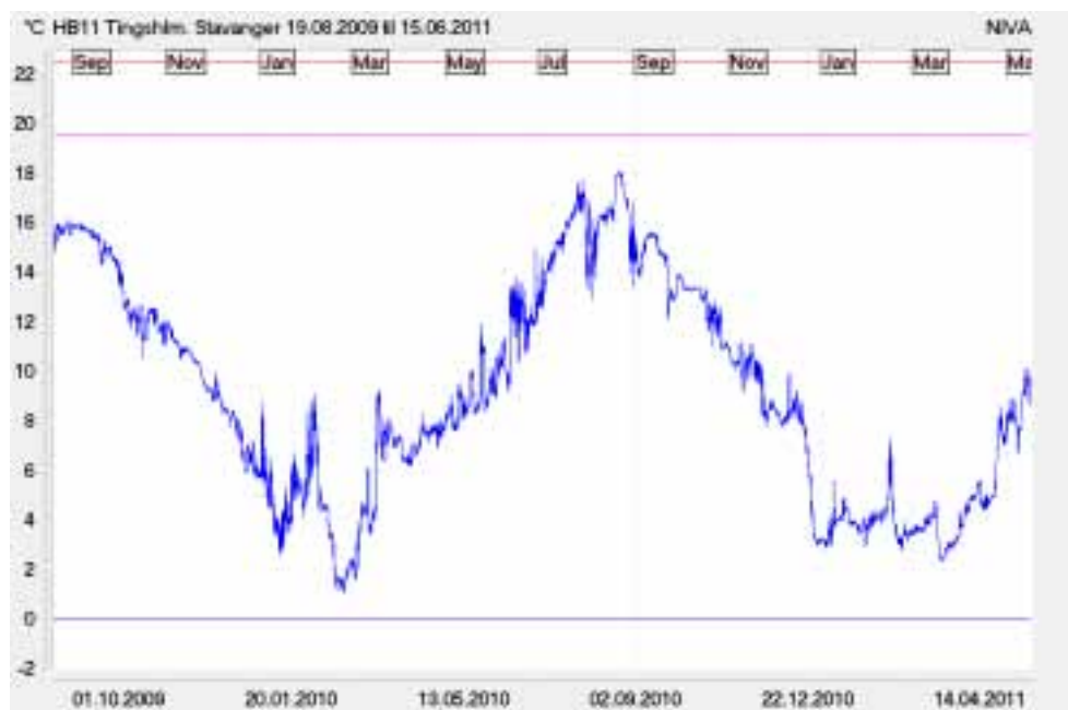
Figur 3.8. Temperaturdata fra 7 meters dyp ved en av dykkerstasjonen HB11 i Hidlefjorden for perioden 19/8-09 til 15/6 2011.
