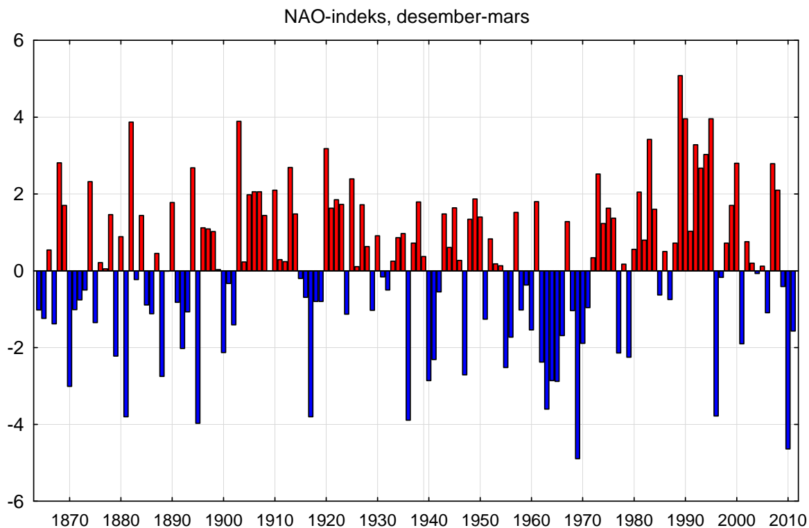
Figur 3.1. North Atlantic Oscillation (NAO) vinterindeks (desember til mars) fra 1864 til 2011 med normalisert lufttrykkforskjell mellom Lisboa, Portugal, og Stykkisholmur/Reykjavik, Island (kilde: http://www.cgd.ucar.edu/cas/jhurrell/indices.html ).
