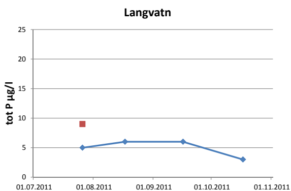
Figur 24. Endringer i total fosfor gjennom sesongen 2011 (blå farge). Til sammenlikning er det lagt inn tidligere data fra 1994 (grønn) (Holtan & Brettum 1996) og 2004 (rød) (Dahl-Hansen 2006).
