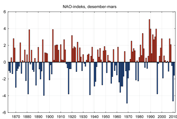
Figur 5. North Atlantic Oscillation (NAO) index fra 1864 til 2011 med middelvei fra desember til mars. (Kilde: http://www.cgd.ucar.edu/cas/jhurrell/indices.html ).
