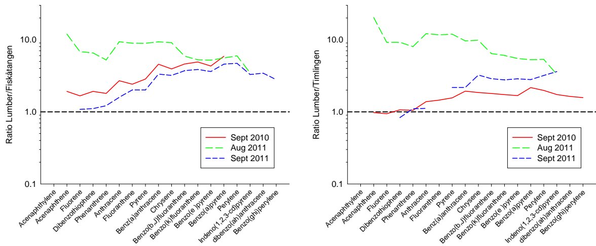
Figur 5. Forholdstall mellom konsentrasjon av PAH målt med SPMD ved Lumber i forhold til Fiskåtangen (venstre) og Lumber i forhold til Timlingen (høyre) i 2010 og 2011. Kun verdier over deteksjonsnivå er plottet.
