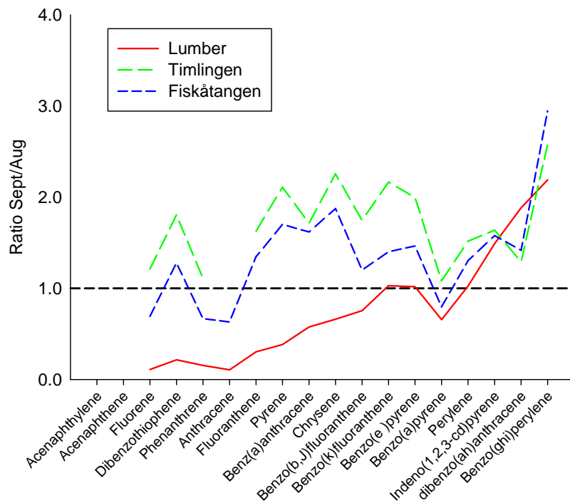
Figur 4. Forholdstall mellom september og august-prøvetakingen i 2011 for PAH-konsentrasjoner målt med SPMD ved Lumber, Timlingen og Fiskåtangen.
