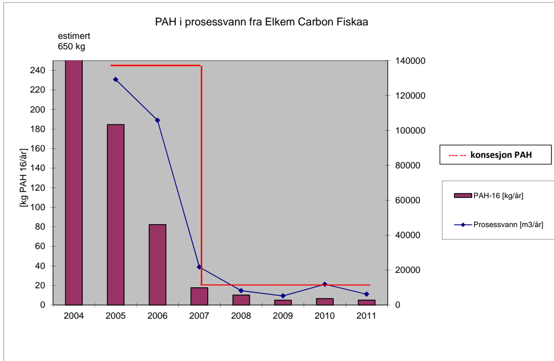
Figur 1. Utslipp av PAH i prosessvann fra Elkem Carbon AS. Data er sammenstilt av Bente Sundby Håland, Elkem Carbon AS.
