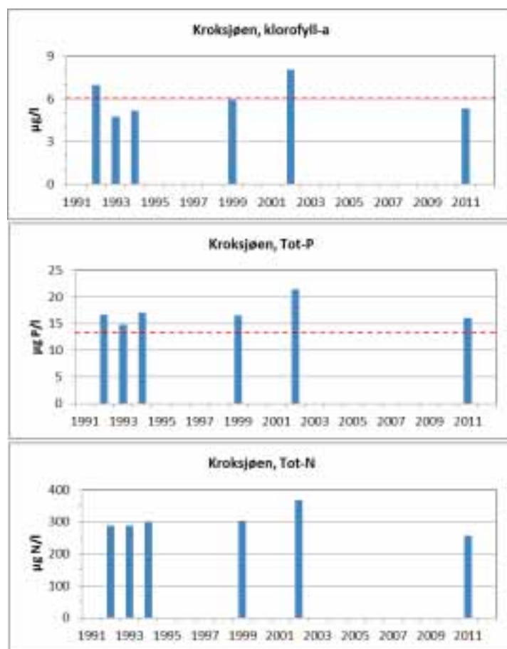
Figur 8. Middelerverdier for klorofyll- a , tot-P og tot-N i Kroksjøen. Røde, stiplede horisontale linjer viser grensene mellom god og moderat tilstand. Kun én observasjon i 2011.
