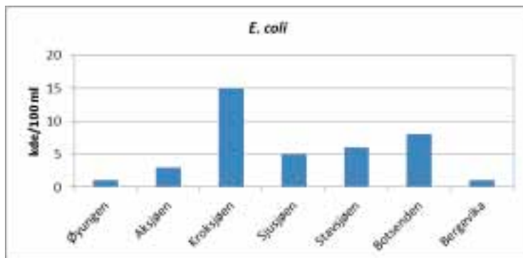
Figur 7. Tetteter av fekale indikatorbakterier (E. coli) den 11.-12. juli 2011.
