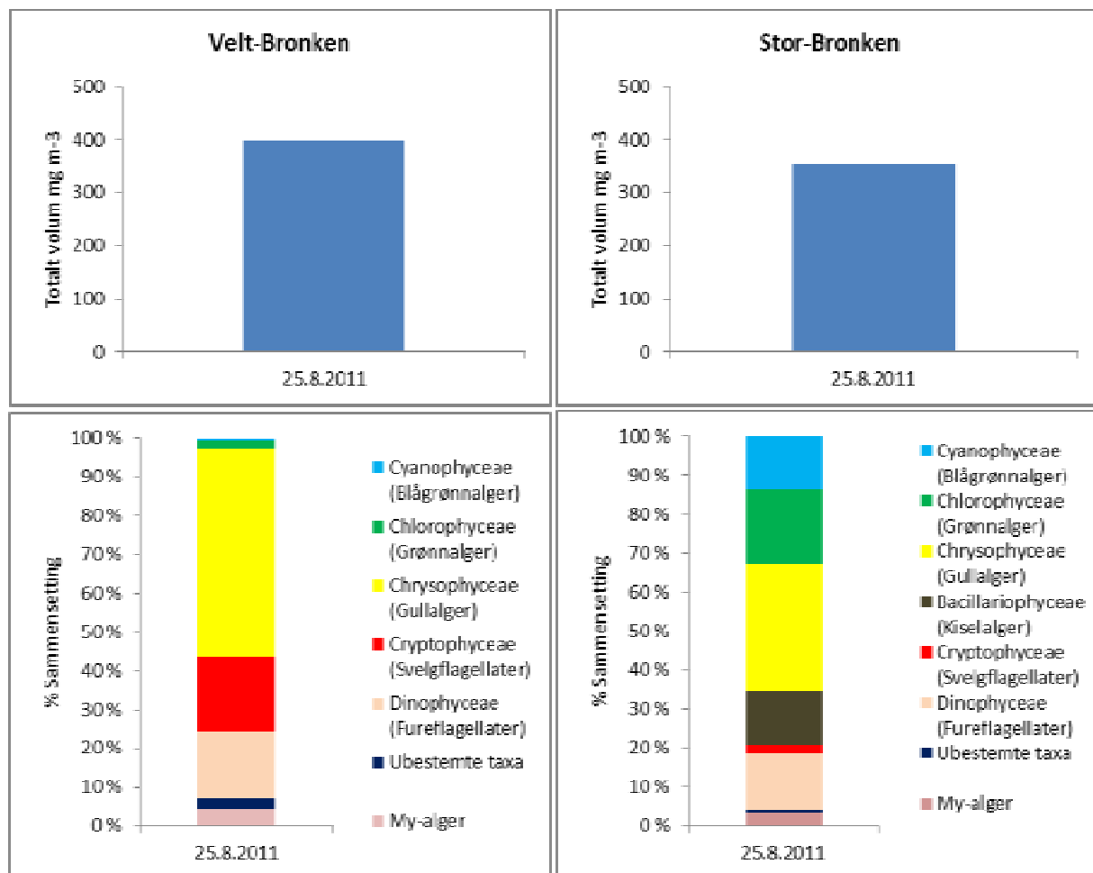
Figur 5. Totalvolumer og prosent sammensetning av hovedgrupper av planteplankton i Velt-Bronken og Stor-Bronken den 25. august 2011.
