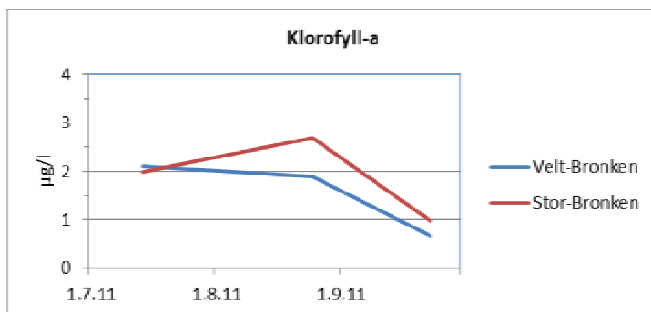
Figur 6. Algemengder målt som klorofyll- a i Velt-Bronken og Stor-Bronken i 2011.
