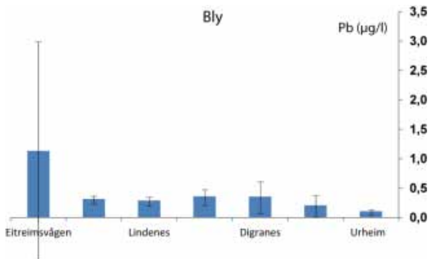
Figur 10. Gjennomsnittskonsentrasjoner av bly (µg/l) i overflatevann i Sørffjorden vist med ± et standardavvik. For Eitrheimsvågen er standardavviket større enn gjennomsnittet.
