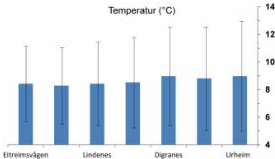
Figur 5. Temperaturvariasjon (årsmiddel og \pm 1 standardavvik) i overflatelaget i Sør fjorden.
