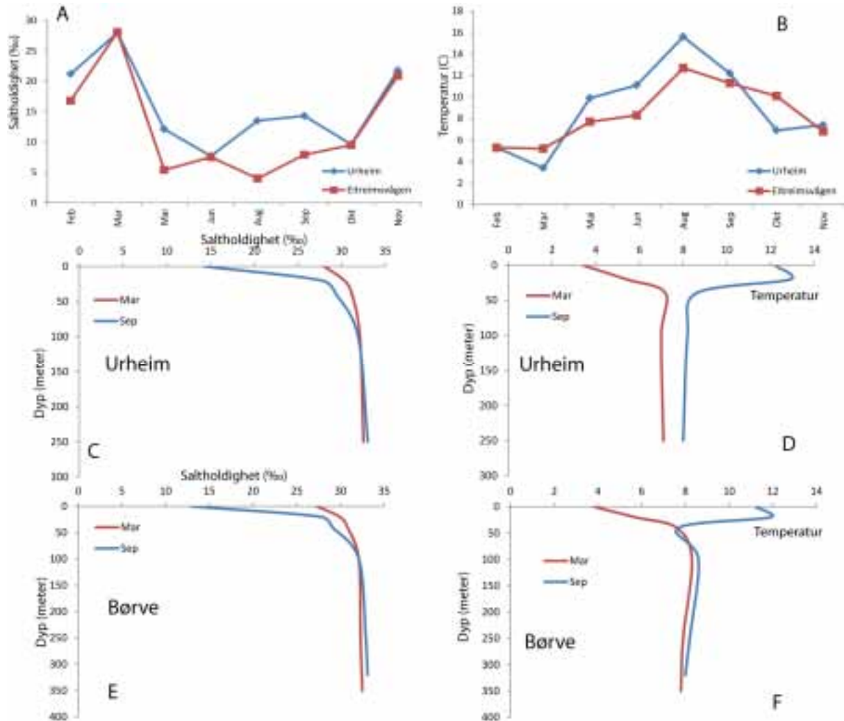
Figur 6. Saltholdighet (A) og temperatur (B) igjennom 2011 ved den innerste og ytterste stasjonen i Sør fjorden (overflaten). Dybdeprofiler for saltholdighet (C) og temperatur (D) ved ytterste (Urheim) og midtre (Børve; hhv. E og F) stasjonen i Sør fjorden. Dybdeprofilene er angitt med glattede kurver basert på 5 og 6 datapunkter per tidspunkt ved hhv. Urheim og Børve.
