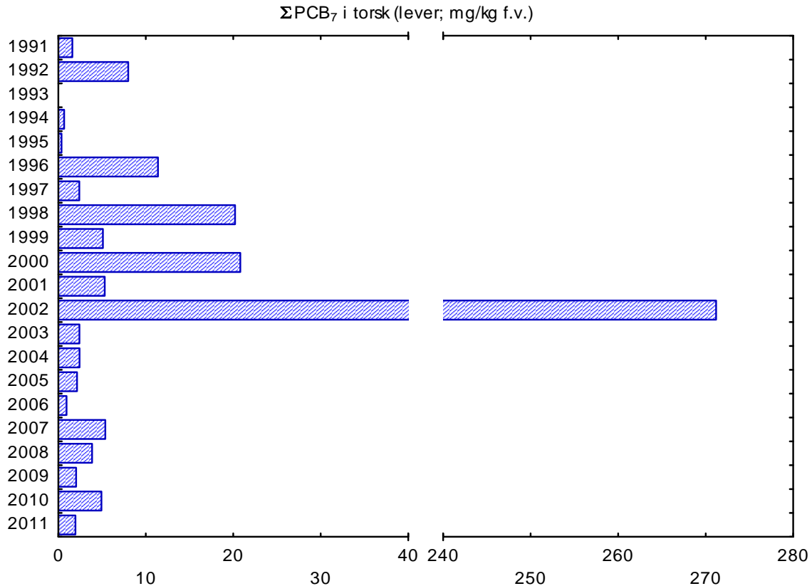
Figur 21. Gjennomsnitt av \Sigma\text{PCB}_7 i lever av torsk fra indre Sør fjorden (1991-2011), mg/kg fettvekt. Verdiene er også gjengitt i Tabell 10. Mrk. brudd på akse mellom 40 og 240.
