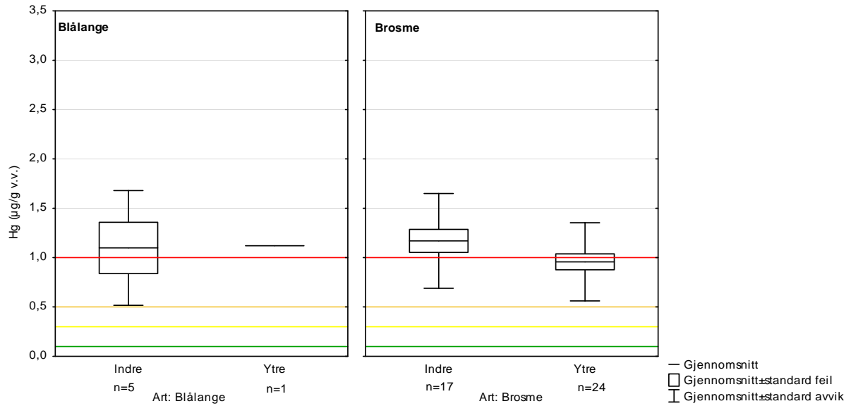
Figur 14. Konsentrasjoner av kvikksølv (mg/kg våtvekt) i dypvannsfisk (blålange, Molva dipterygia ; brosme, Brosme brosme ) fra Sørkjøya (indre og ytre fjord; antall analyserte prøver angitt) i 2011. Til sammenligning er nedre grenser for Klifs tilstandsklasser for kvikksølv i filet av torsk også angitt (grønn: Kl. II; gul: Kl. III; oransje: Kl. IV; rød: Kl. V).
