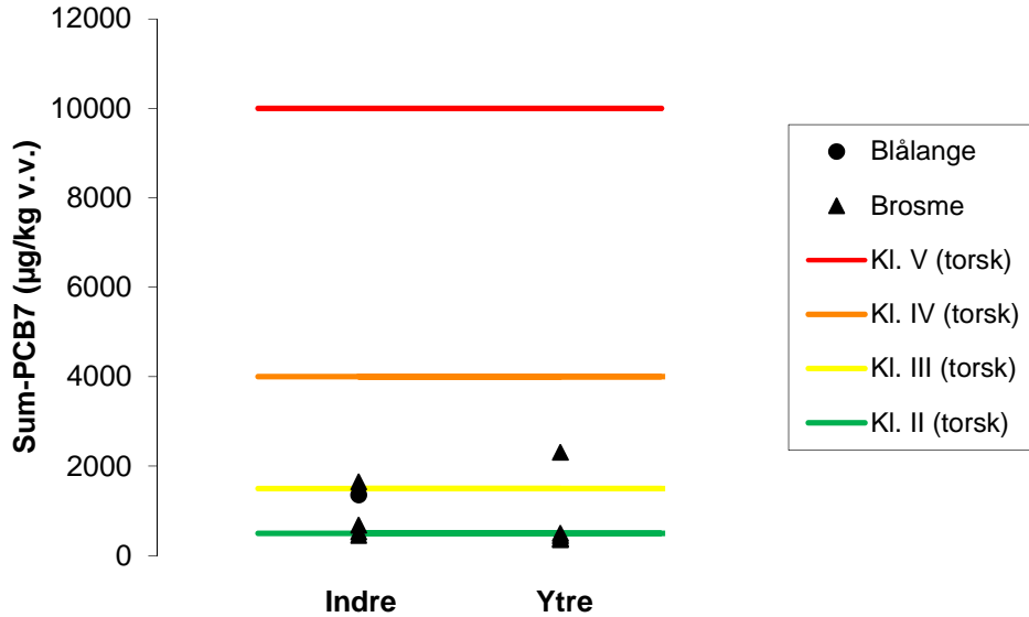
Figur 23. Konsentrasjoner av \Sigma\text{PCB}_7 ( \mu\text{g}/\text{kg} våtvekt) i lever av dypvannsfisk (blålange, Molva dipterygia ; brosme, Brosme brosme ) fra Sør fjorden (indre og ytre fjord) i 2011. Til sammenligning er nedre grenser for Klifs tilstandsklasser for \Sigma\text{PCB}_7 i lever av torsk angitt. For blandprøvenes sammensetning se Vedlegg.
