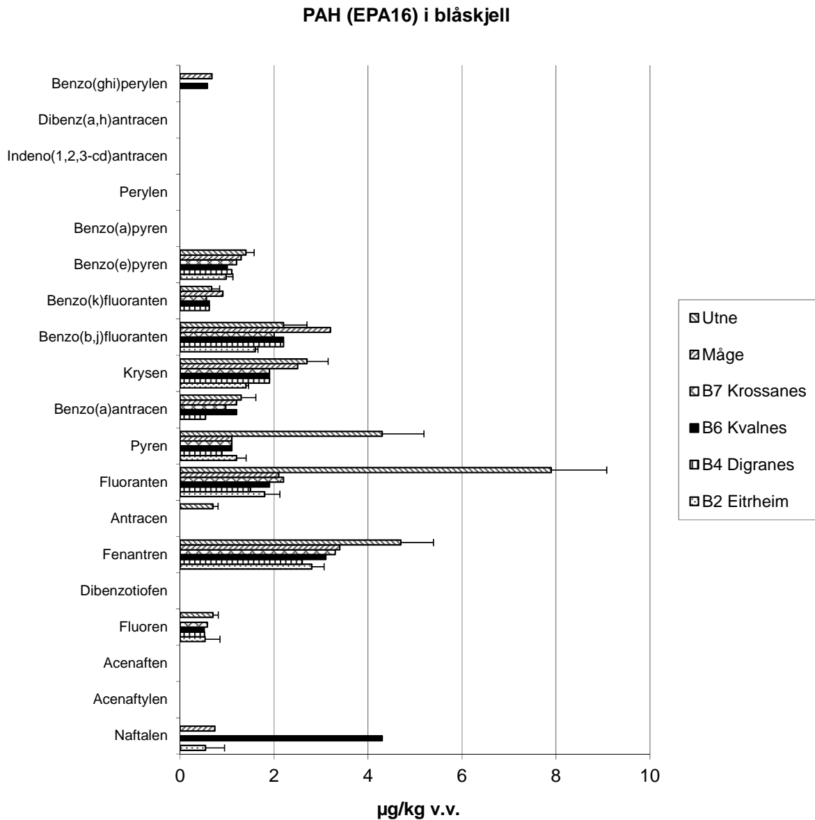
Figur 27. Konsentrasjoner ( \mu\text{g}/\text{kg} våtvekt) av polysykliske aromatiske hydrokarboner (PAH) i blåskjell fra stasjonsnettet i Sørffjorden, 2011. Median av 3 replikater på stasjon B2 (Eitrheim) og stasjon "Utne". Standard avvik er angitt for disse.
