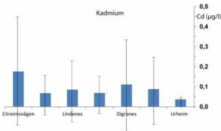
Figur 9. Gjennomsnittlige kadmiumkonsentrasjoner ( \mu\text{g/l} ) vist med \pm et standardavvik for overflateprøver fra Sør fjorden. På grunn av høye konsentrasjoner i februar er alle standardavvikene store.
