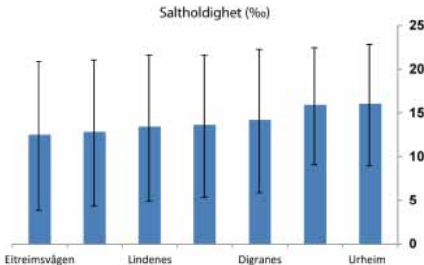
Figur 4. Saltholdighet (‰, årsmiddel og \pm 1 standardavvik) i overflatevannet i Sørffjorden i 2011. Venstre er sørvest og høyre nordøst i fjorden.
