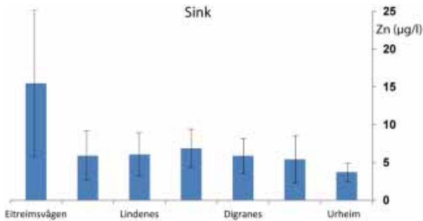
Figur 8. Gjennomsnittlige konsentrasjoner av sink ( \mu\text{g/l} ) vist \pm et standardavvik for overflateprøver fra Sør fjorden i 2011.
