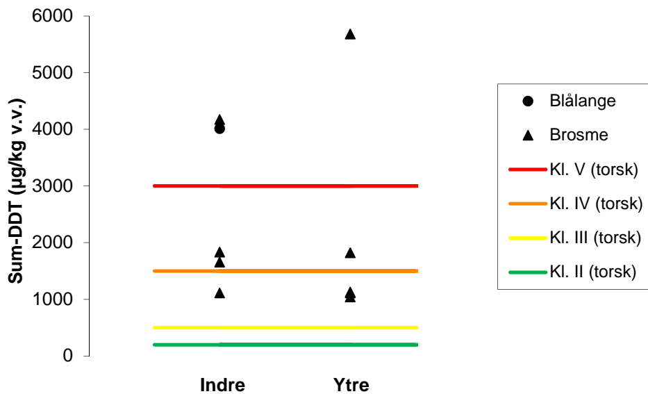
Figur 24. Konsentrasjoner av \Sigma\text{DDT} ( \mu\text{g}/\text{kg} våtvekt) i lever av dypvannsfisk (blålange, Molva dipterygia ; brosme, Brosme brosme ) fra Sør fjorden (indre og ytre fjord) i 2011. Til sammenligning er nedre grenser for Klifs tilstandsklasser for \Sigma\text{DDT} i lever av torsk angitt. For blandprøvenes sammensetning se Vedlegg.
