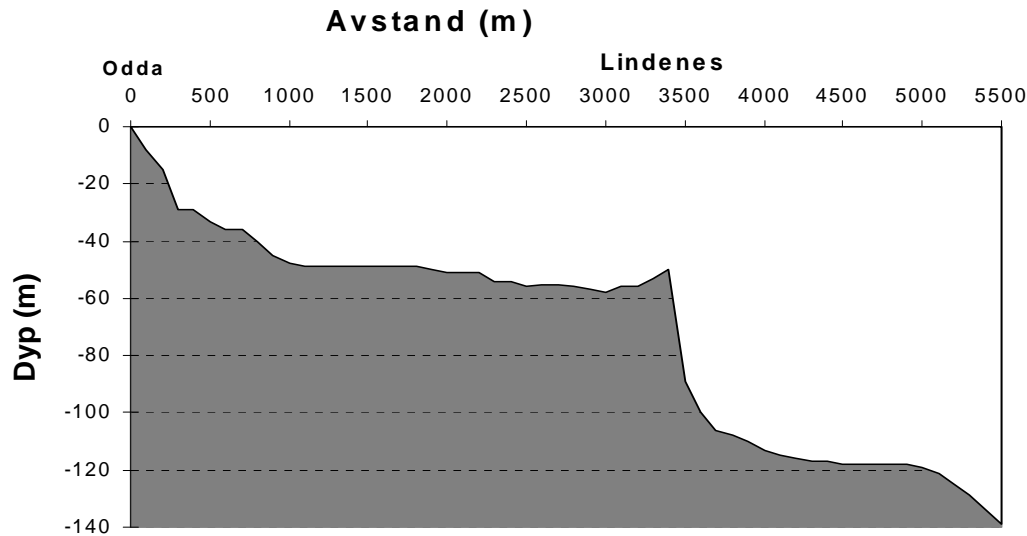
Figur 2. Langsgående bunnprofil fra Odda til Tyssedal. Indre del av Sjørfjorden har ingen terskel av betydning som kan hindre vannutskiftingen.
