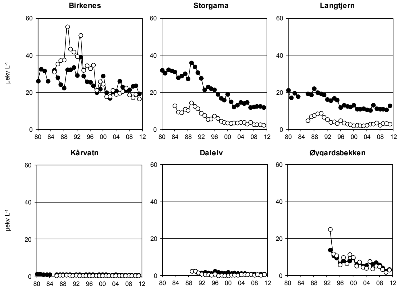
Figur 39. \text{H}^+ og labilt Al i feltforskningsstasjonene. \text{H}^+ ● og labilt Al ○. Enhet: \mu\text{ekv L}^{-1} .
