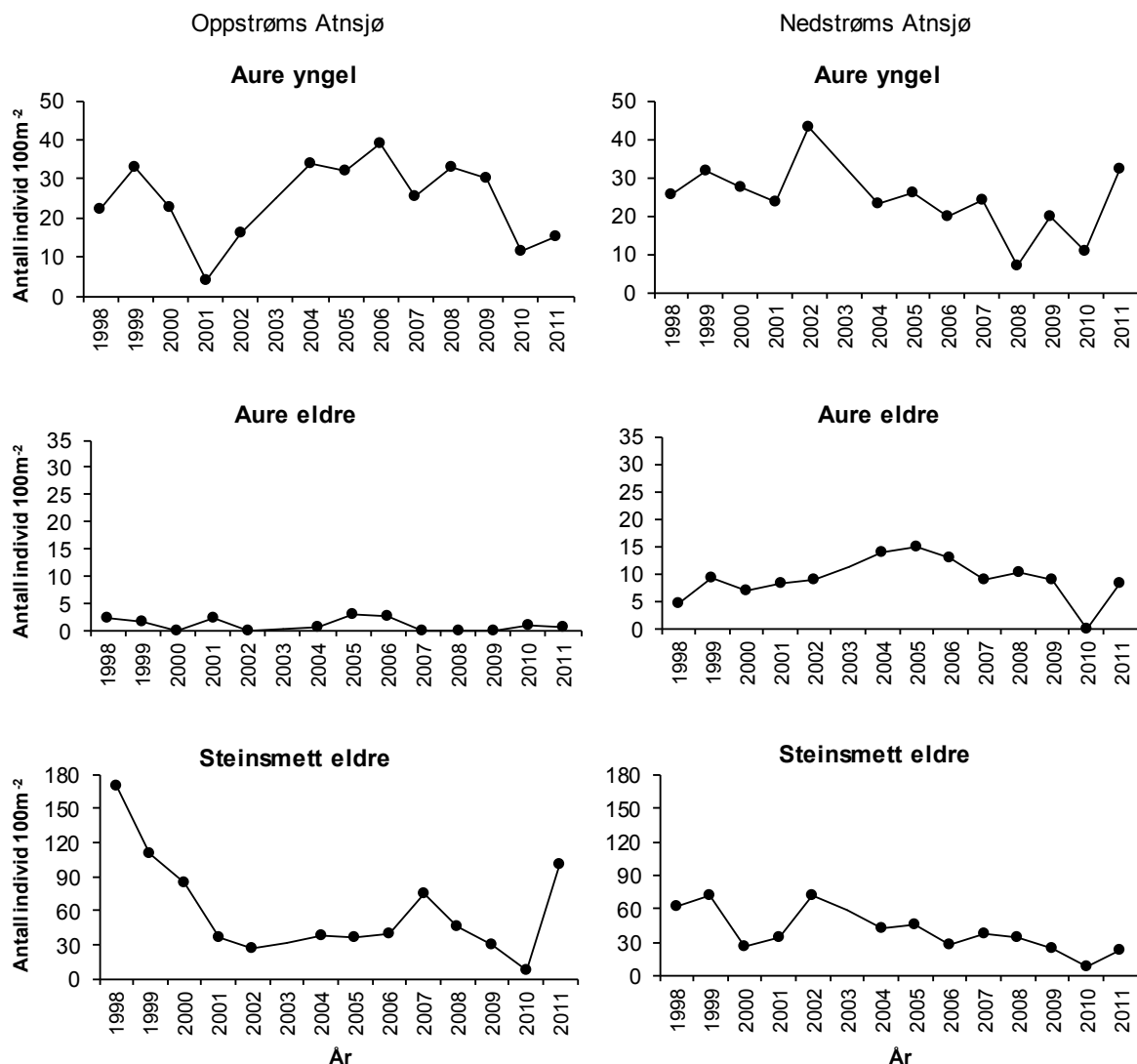
Figur 72. Tettheten av fisk pr.100 m 2 i Atna på stasjoner oppstrøms og nedstrøms Atnsjøen, fordelt på yngel (0+) og eldre individ ( \geq 1+ ) av aure og eldre individ ( \geq 1+ ) av steinsmett i perioden 1998-2011. I 2003 ble det ikke samlet inn fisk.
