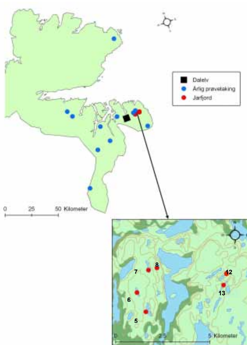
Figur 25. Lokalisering av overvåkingslokaliteter i Øst-Finnmark, i Sør-Varanger kommune. Både Jarfjordfjell-sjøene, tidstrendsjøene (årlig prøvetaking) og feltforskningsstasjonen Dalelv er vist på kartet. Tallene er en forkortelse av identifikasjonen på lokalitetene (5 er JAR-05, 6 er JAR-06 osv.).
