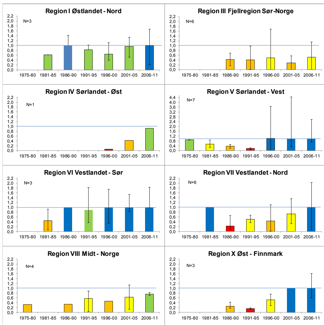
Figur 64. Utviklingen i tilstandsklasser av mulig forsuringsskadede aurebestander i femårs perioder, basert på fem klasser som angitt i Tabell 15. Blå: svært god, Grønn: god, Gul: moderat, Oransje: dårlig og Rød: svært dårlig. Vertikale stolper angir minimum- og maksimumsverdi. N = antall innsjøer som omfattes av beregningene.
