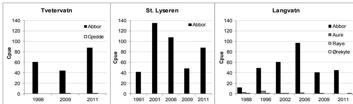
Figur 46. Fangst av abbor og gjedde pr. 100 m 2 bunngarnareal på 0-6 m dyp (Cpue) i Tvetervatn, av abbor i St. Lyseren, og av abbor, aure, røye og ørekyte i Langvatn i ulike perioder fra 1988 til 2011.
