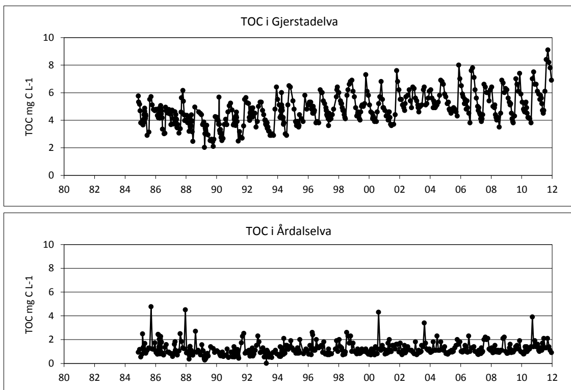
Figur 34. Total organisk karbon (TOC) i Gjerstadelva og Årdalselva for perioden 1980 - 2011. Enhet \text{mg C L}^{-1} .
