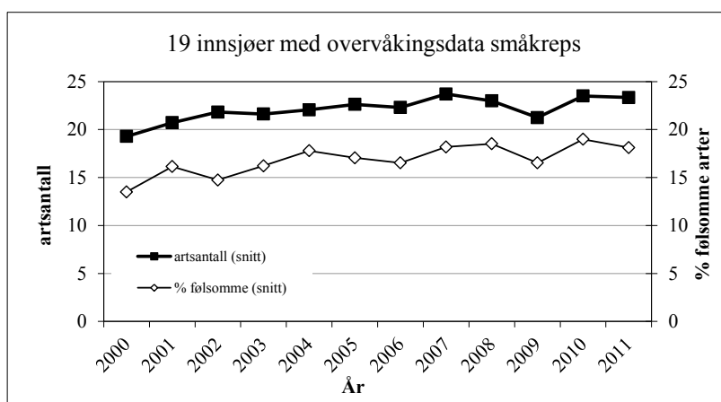
Figur 63. Gjennomsnittlig antall arter av småkreps ( Cladocera + Copepoda ) og andel forsureningsfølsomme småkreps (% av totalt antall arter) for 19 innsjøer med årlige undersøkelser i perioden 2000-2011.
