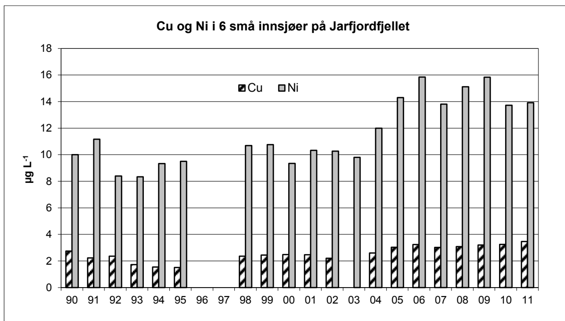
Figur 27. Årlige middeler verdier for kobber og nikkel i seks små innsjøer på Jarfjordfjellet fra 1990 til 2011.
