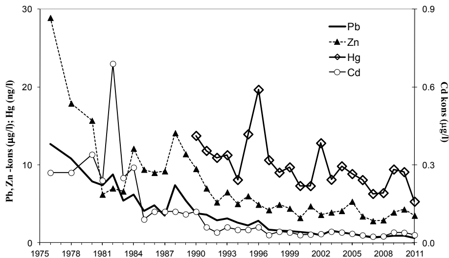
Figur 7. Middelt konsentrasjonene av bly, kadmium og sink i nedbør på Birkenes, Aust-Agder for årene 1976-2011. For kvikk sølv er målingene fra 1990-2003 fra Lista.
