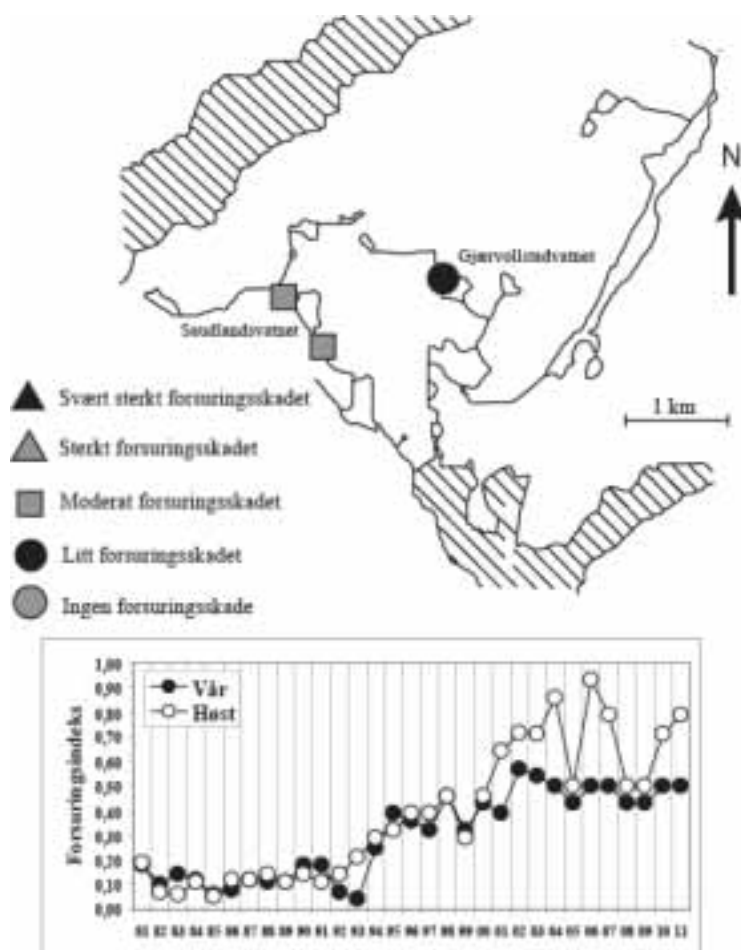
Figur 67. Oversikt over innsamlingslokaliteter og sammensetning av bunndyr i Farsundområdet i 2011. Figuren viser også gjennomsnittlige foruringsverdier vår (V) og høst (H) i perioden 1981-2011.
