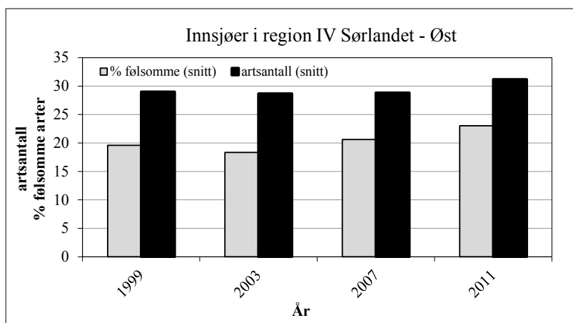
Figur 48. Gjennomsnittlig antall arter av småkreps ( Cladocera + Copepoda ) og andel forsurningsfølsomme småkreps (% av totalt antall arter) for 6 innsjøer i region IV (Sørlandet – Øst) undersøkt i 1999, 2003, 2007 og 2011.
