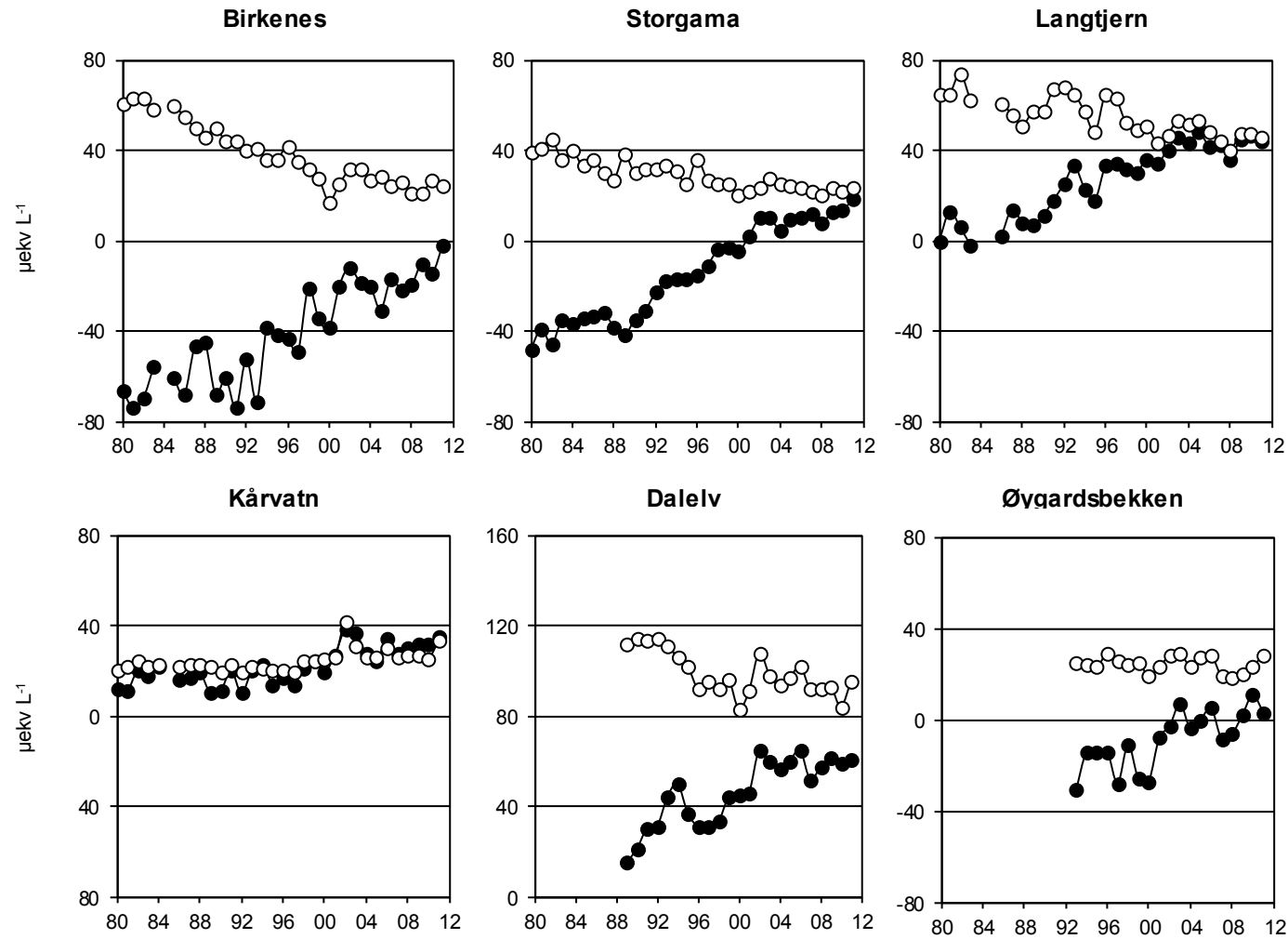
Figur 38. ANC og ikke-marine basekationer ( \text{Ca}+\text{Mg} ) i feltforskningsstasjonene. ANC \bullet og ikke-marine basekationer ( \text{Ca}+\text{Mg} ) \circ . Enhet: \mu\text{ekv L}^{-1} . OBS! Skala Dalelva.
