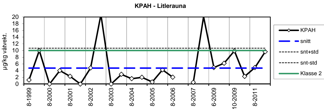
Figur 5. Utvikling i KPAH-innholdet i strandsnegl ved de fire stasjonene på Lista fra 1999-2011. Grensene for SFTs tilstandsklasser (for blåskjell) er vist som farget, heltrukket linje. Fargen er i hht. tilstandsklassen. Stiplede blå linjer viser snittverdier for hele perioden (1999-2011) for den enkelte stasjon. Stiplede sorte linjer viser standardavvik. NB! Alle grafene har ulik skala.
