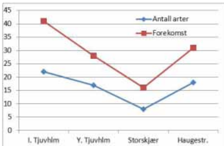
Figur 17. Artsantall og forekomst (mengde) på 4 stasjoner i Husebybukta 2011.
