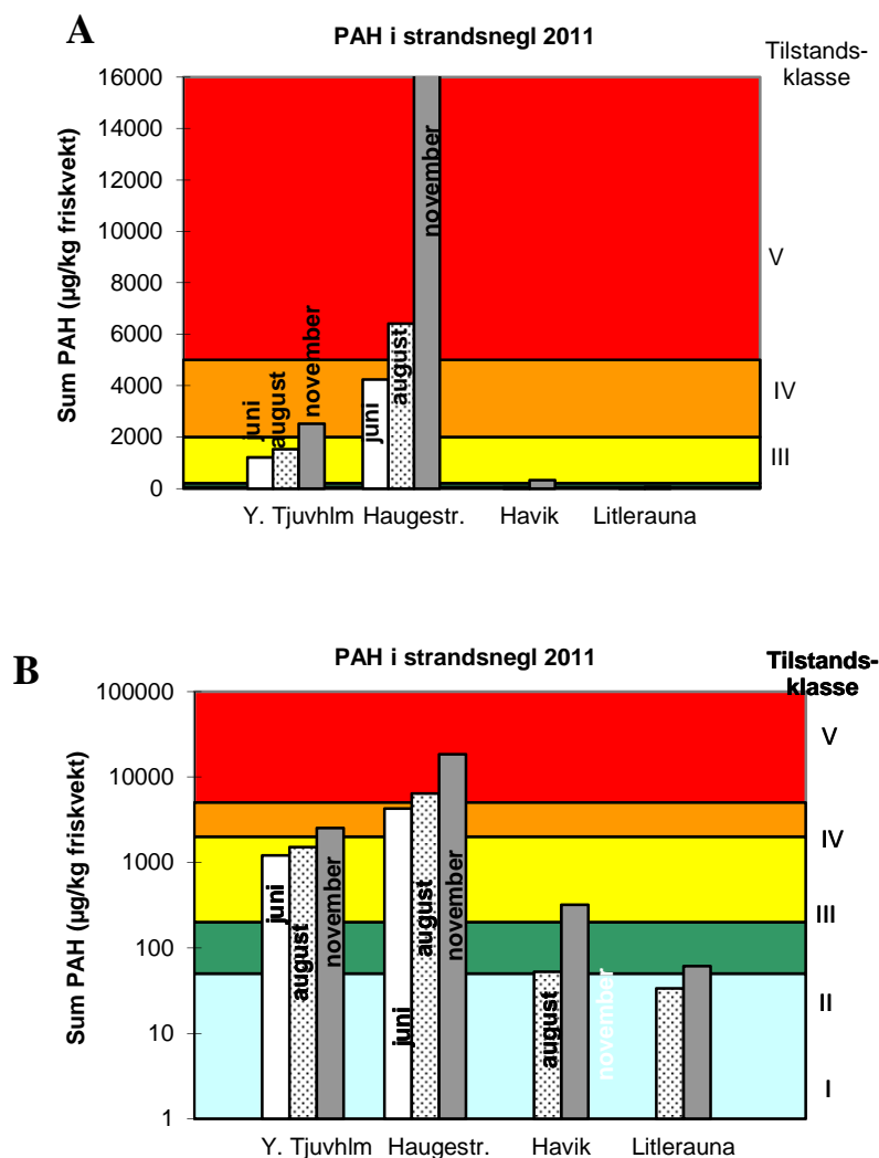
Figur 3. PAH i strandsnegl fra fire stasjoner på lista i 2011. Verdiene er oppgitt som PAH 16 i µg/kg friskvekt. Farge angir tilstandsklasse i hht. SFTs klassifiseringssystem. Grafe A viser nivåene på vanlig skala. Grafe B viser nivåene på logaritmisk skala for å synliggjøre referansestasjonene.
