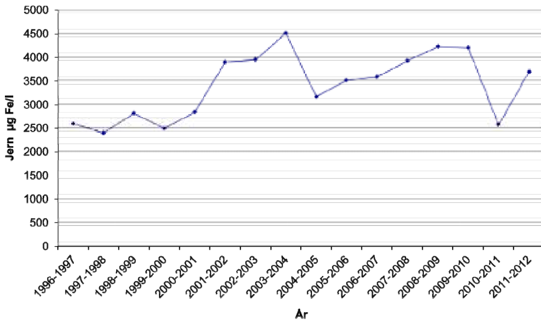
Figur 6. Tidsveide årsmiddelverdier for jern i Orva. Hydrologiske år 1996-2012.
