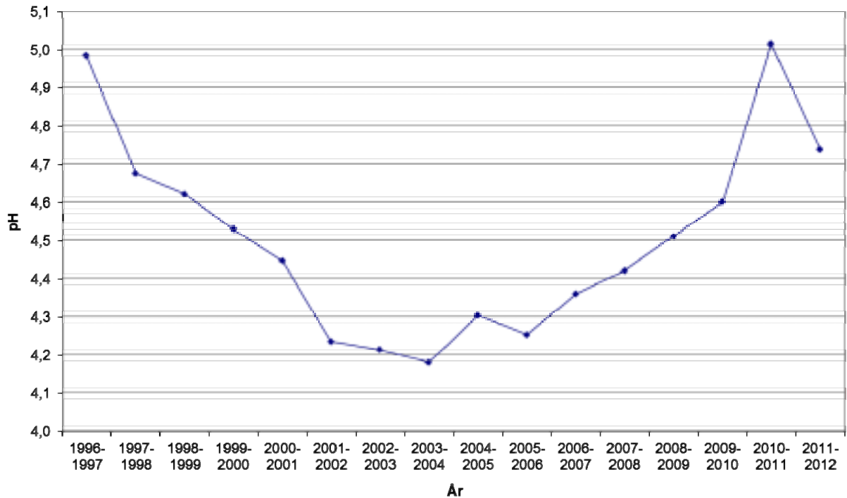
Figur 5. Tidsveide årsmiddelverdier for pH. Hydrologiske år 1996-2012.
