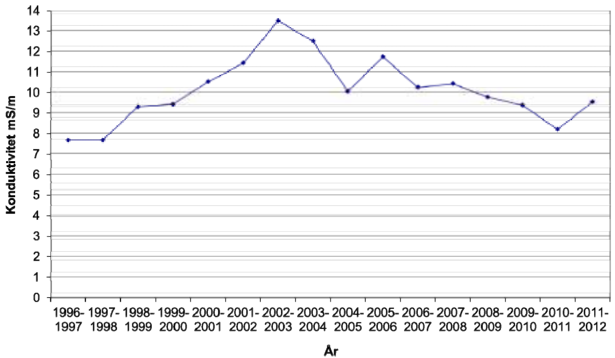
Figur 8. Tidsveiede årsmiddelverdier for konduktivitet i Orva. Hydrologiske år 1996-2012.
