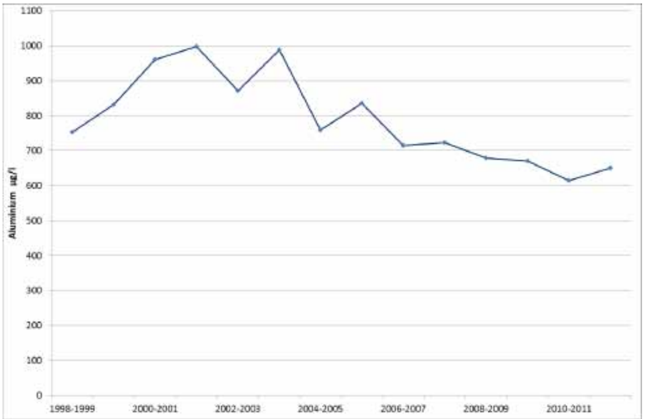
Figur 10. Tidsveiede årsmiddelverdier for aluminium i Orva. Hydrologiske år 1996-2012.
