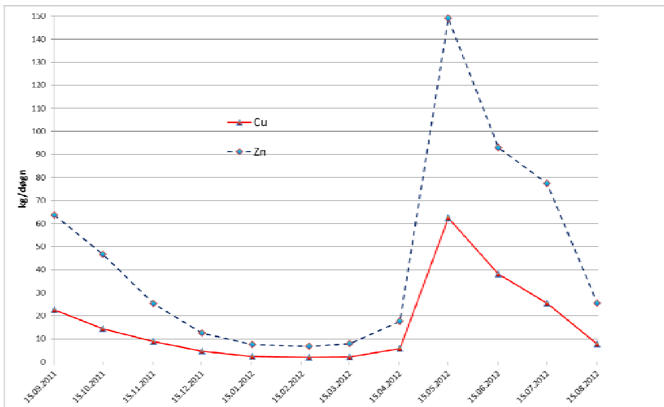
Figur 11. Øyeblikkstransport av kobber og sink i 2011-2012.
