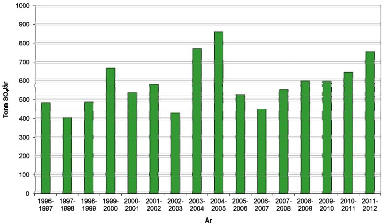
Figur 14. Transport av sulfat i Orva. Hydrologiske år.
