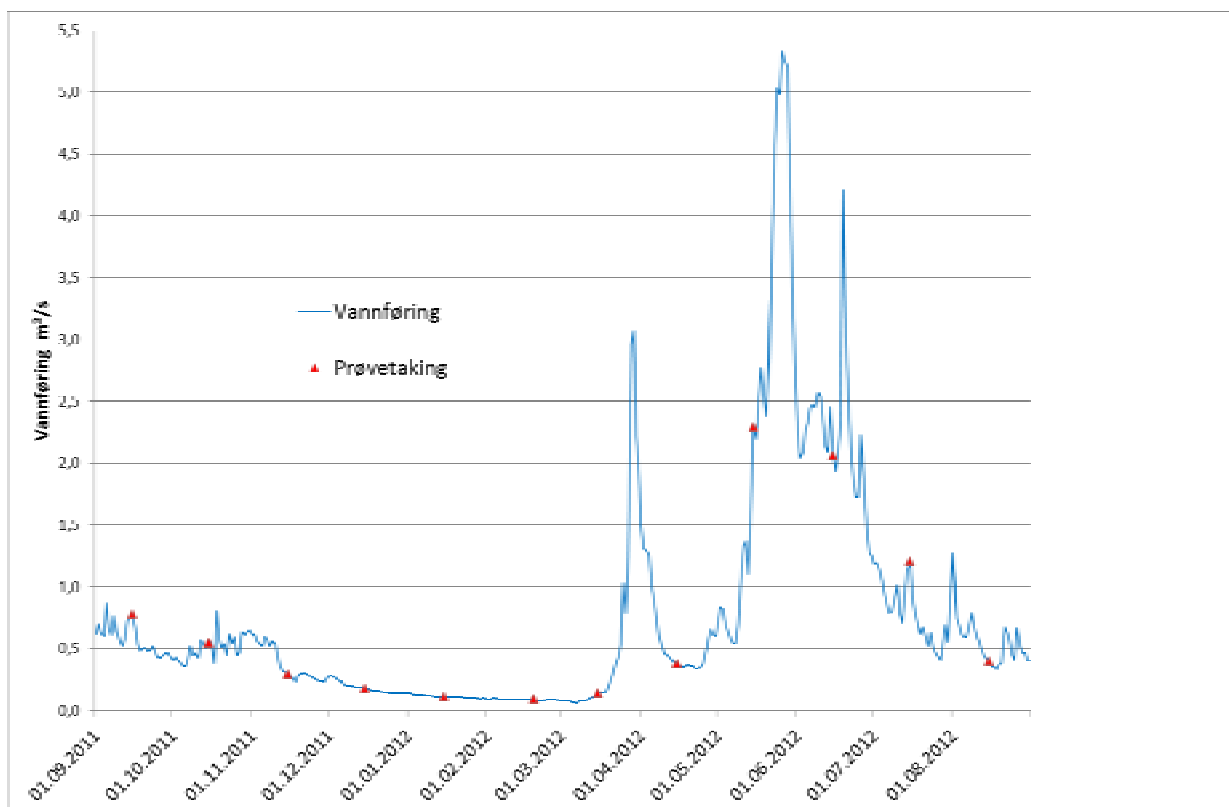
Figur 4. Døgnmiddelvannføringer i Orva ved Litlstugguvollen i 2011-2012 med markering av prøvetakingstidspunkter.
