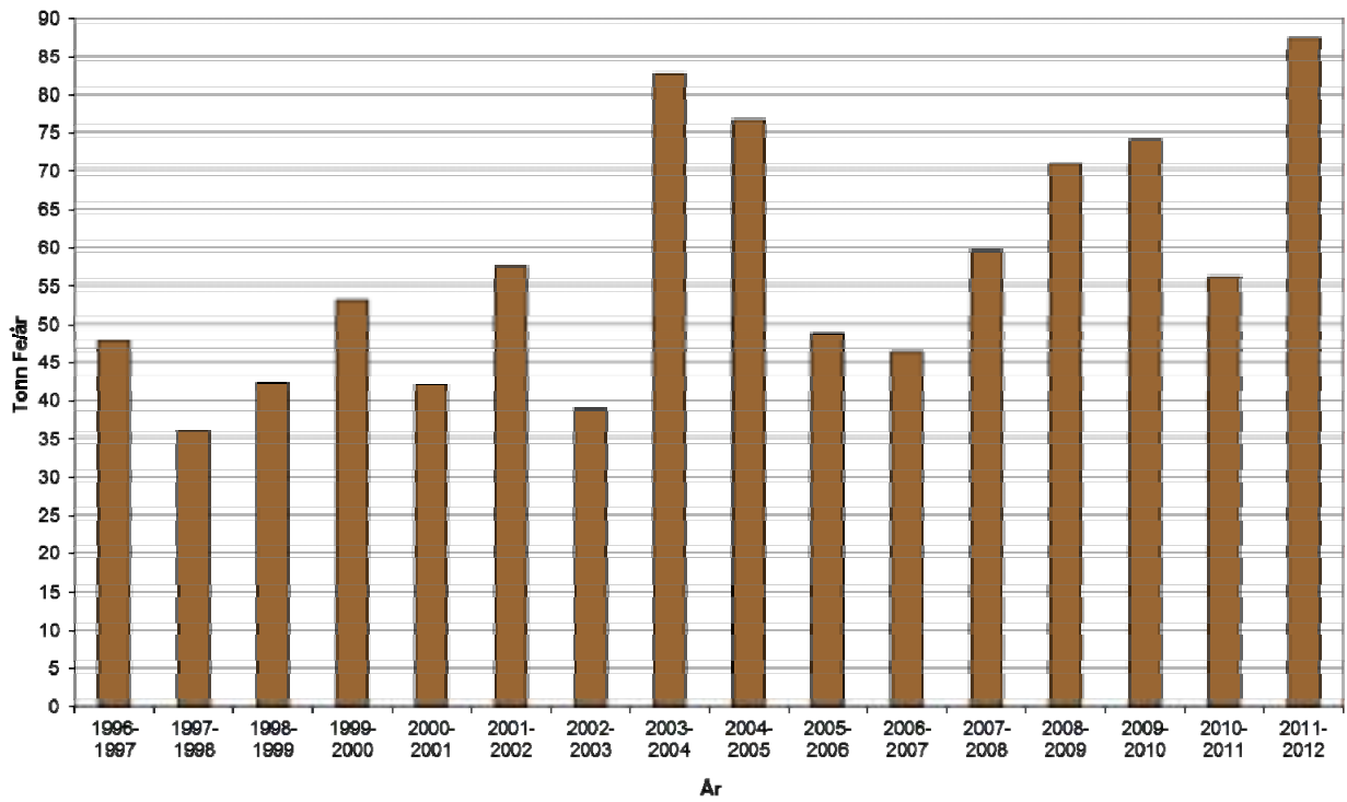
Figur 13. Transport av jern i Orva. Hydrologiske år.
