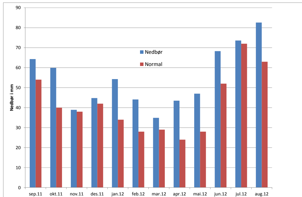
Figur 3. Månedlige nedbørhøyder og normaler i året 2011-2012.
