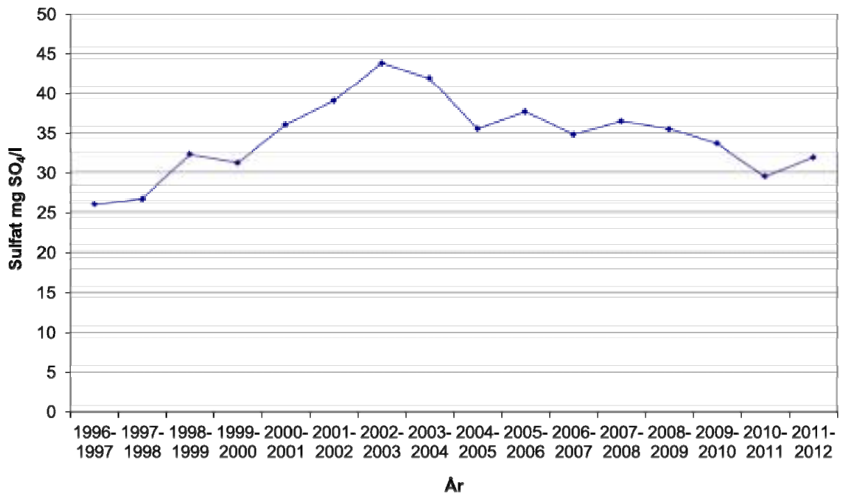
Figur 9. Tidsveiede årsmiddelverdier for sulfat i Orva. Hydrologiske år 1996-2012.
