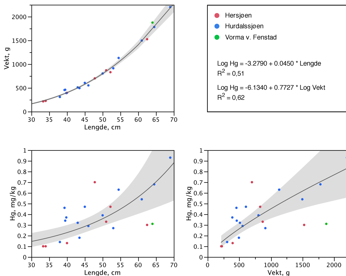
Figur 6. Forholdet mellom fiskelengde og vekt (a); fiskelengde og kvikksølv (b); fiskevekt og kvikksølvkonsentrasjon (Hg, mg/kg) for gjedde fra vannområde Hurdalssjøen/Vormå, fisket i 1989/1990. Båndet omkring regresjonene er 95 % konfidensgrense. Regresjonene for kvikksølv (log-transformert) mot fiskestørrelse er gitt i øvre høyre panel.
