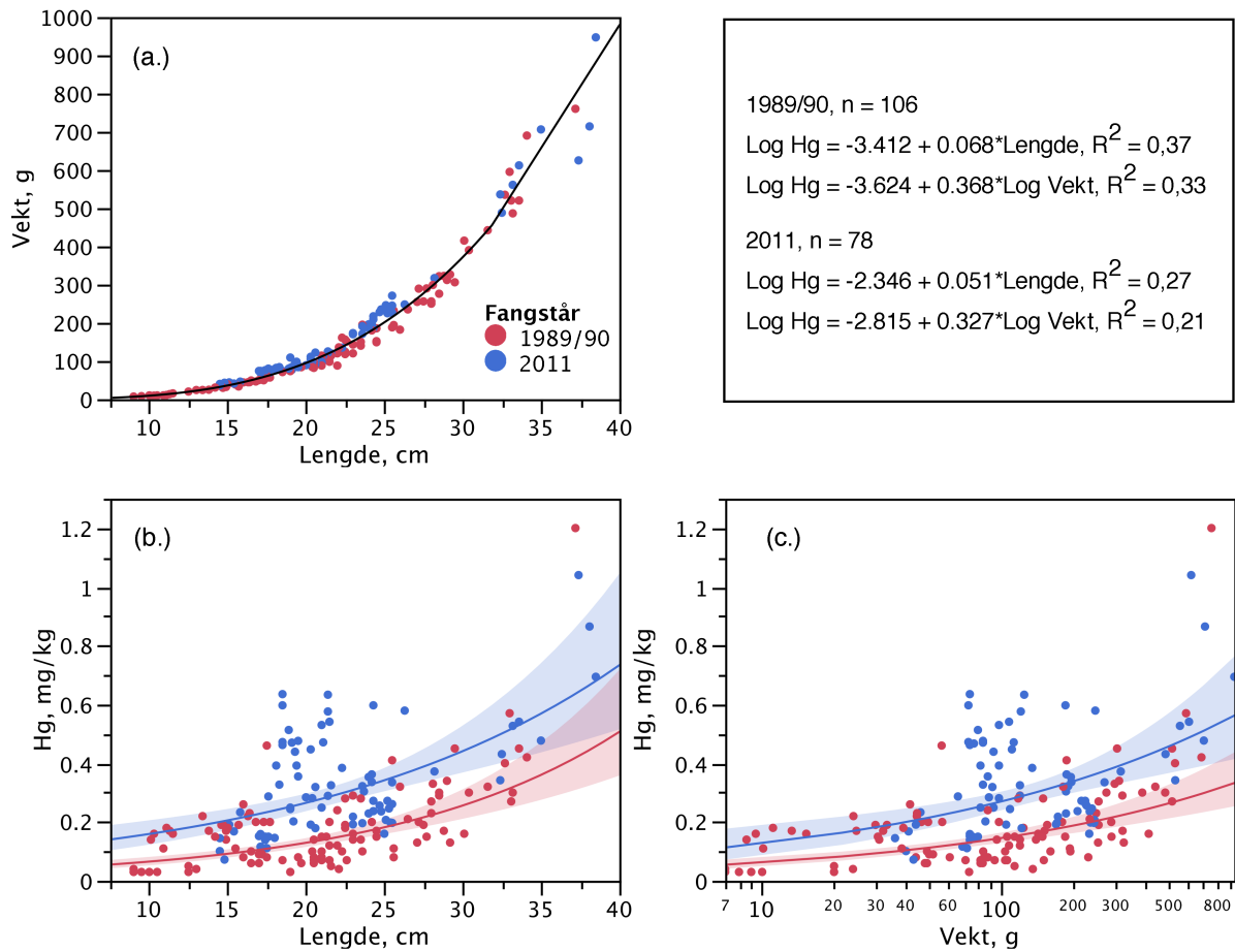
Figur 4. Forholdet mellom fiskelengde og vekt (a); fiskelengde og kvikksølv (b); fiskevekt og kvikksølvkonsentrasjon (Hg, mg/kg) i lokalitetene (c) fra vannområde Hurdalsvassdraget/Vorma. Regresjonene for kvikksølv (log-transformert) mot fiskestørrelse er gitt i øvre høyre panel.
