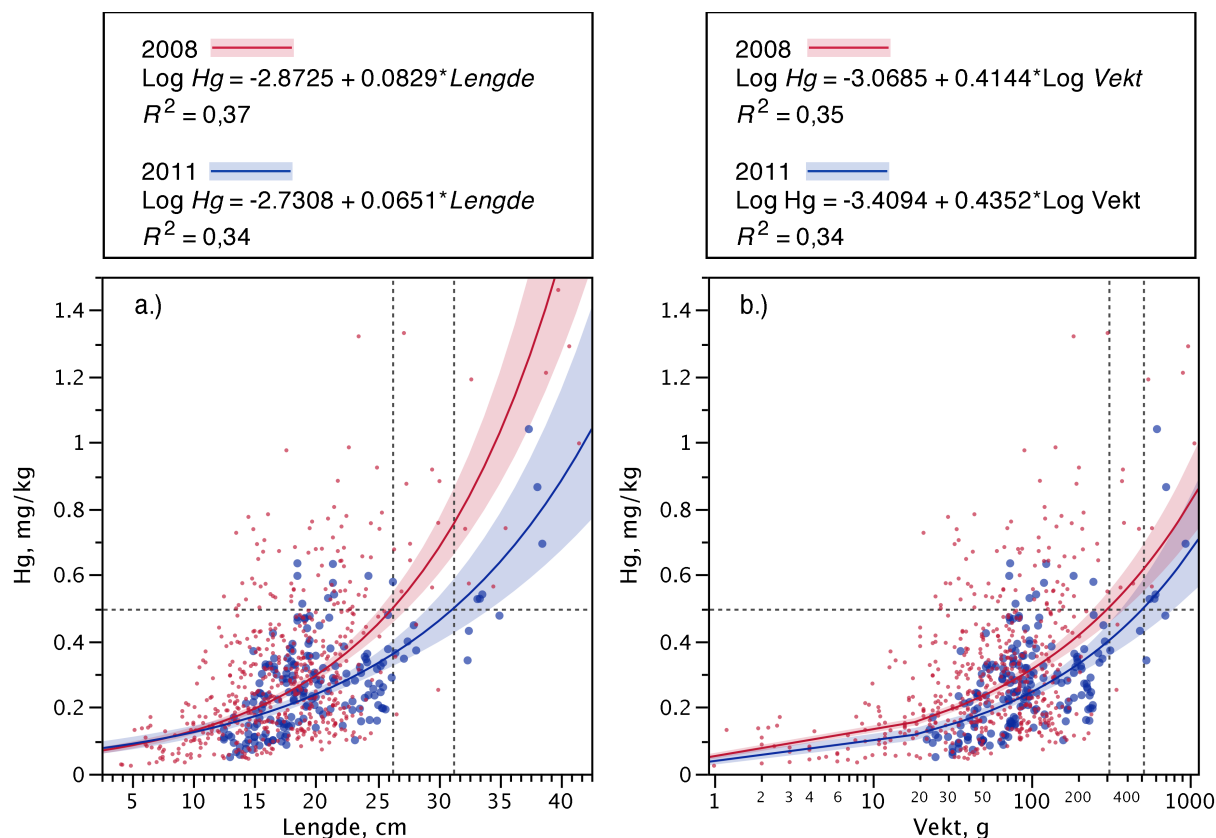
Figur 7. Forholdet mellom kvikksølvkonsentrasjon i abbor (Hg, mg/kg) og (a.) fiskelengde og (b.) fiskevekt fra foreliggende undersøkelse (2011, n = 187) og en regional undersøkelse fra Sør-Norge (2008, n = 565). Regresjonene for kvikksølv (log-transformert) mot fiskestørrelse er gitt i panelene over grafene. Båndet omkring regresjonene er 95 % konfidensgrense. De stiplede linjene viser omsetningsgrensen (0,5 mg Hg/kg) og de beregnede korresponderende fiskestørrelser.
