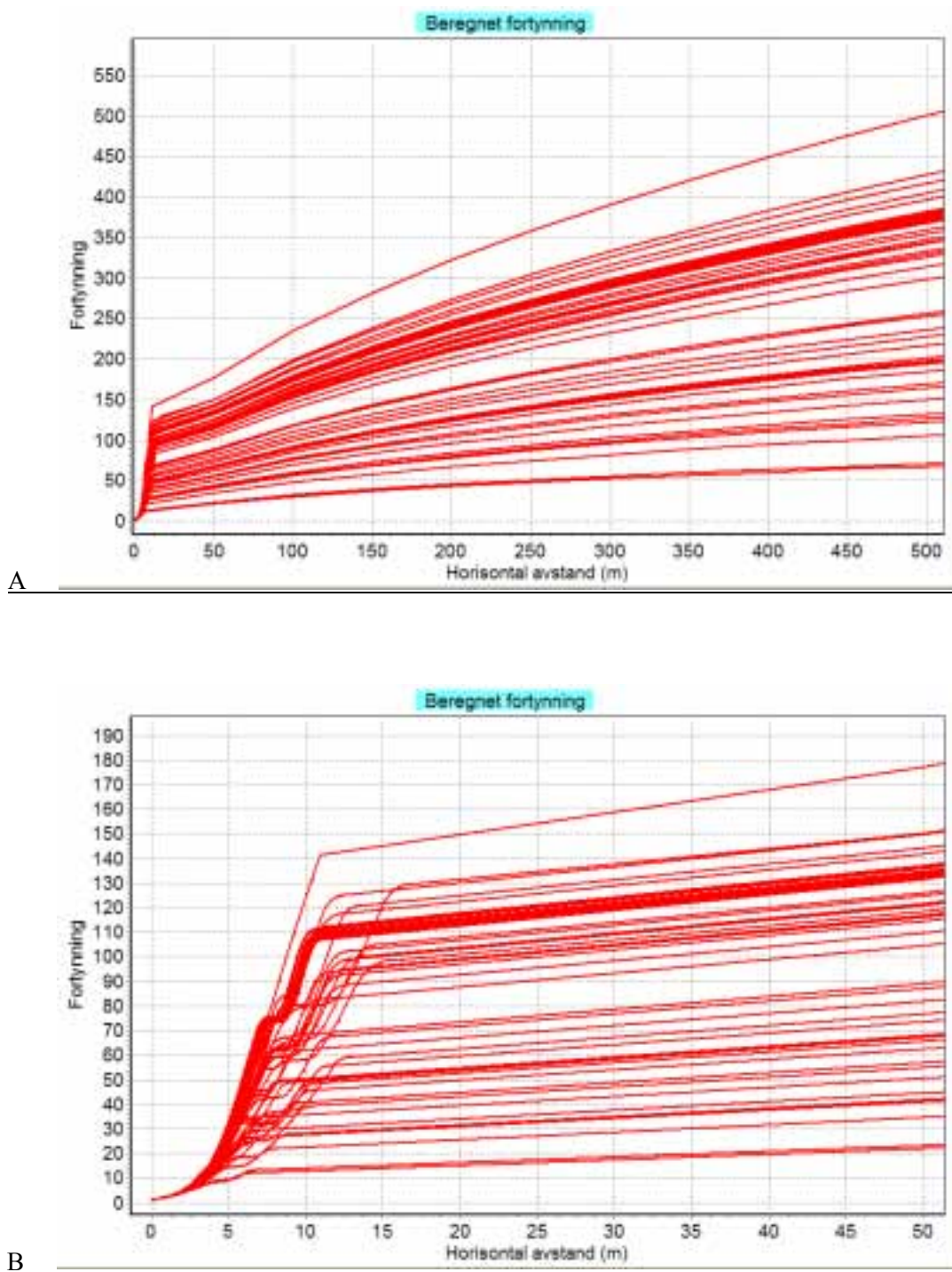
Figur 4. Beregnet fortyning av avløpsvannet for de 50 simulerte situasjoner ved en strømhastighet på 3 cm/s. A: Resultatet for 0-500 m. B: Resultatet for 0-50 m. Data fra (Schaanning and Næs 2006).
