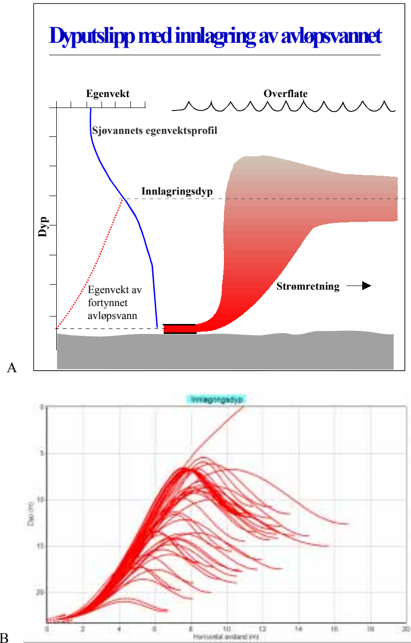
Figur 3. A. Prinsippskisse som viser hvordan et dyputslipp av avløpsvann fungerer i forhold til innlagring. En forutsetning for innlagring er at egenvekten for fjordvannet øker med dyppet (vertikal stabil sjiktning). B. Simulering av innlagringsdyp for utslippsvannet ved utslipp i 23 m dyp. Data fra (Schaanning and Næs 2006).
