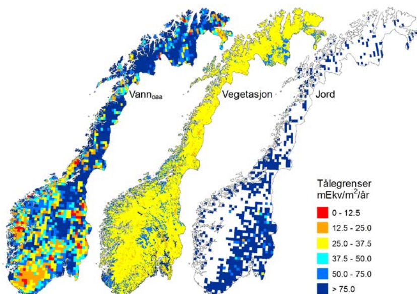
Figur 1. Tålegrenser for vann (organiske syrer inkludert), vegetasjon og jord i Norge.
