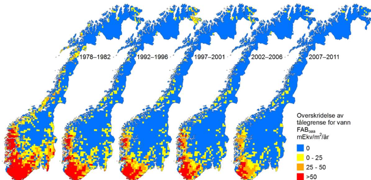
Figur 4. Beregnet overskridelse av tålegrenser for forsurening av overflatevann med bruk av FAB_{\text{aaa}} -modellen.
