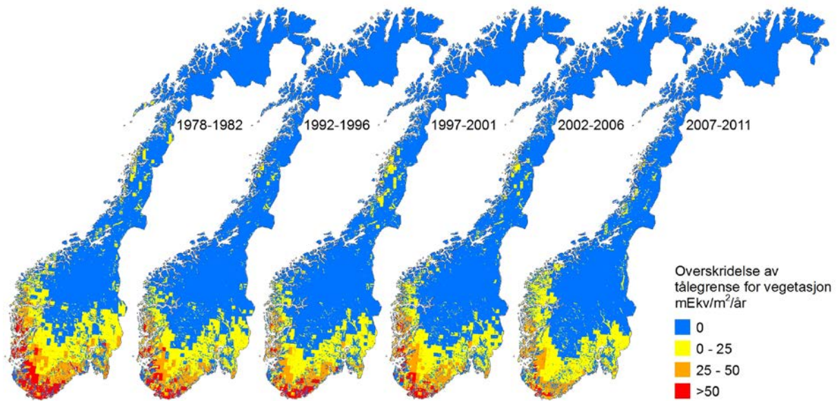
Figur 5. Beregnet overskridelse av tålegrenser for overgjødslingseffekter av vegetasjon (empiriske tålegrenser).
