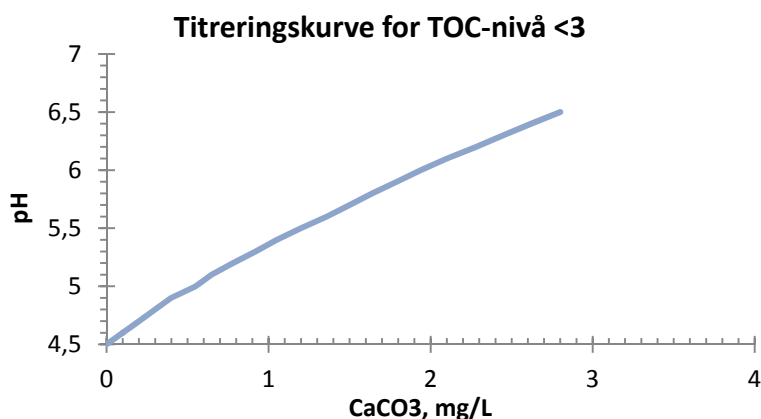
Figur 5. Titreringskurve for TOC-nivå <3 mg/l, gir CaCO 3 behov (mg/L) ved ulik pH
