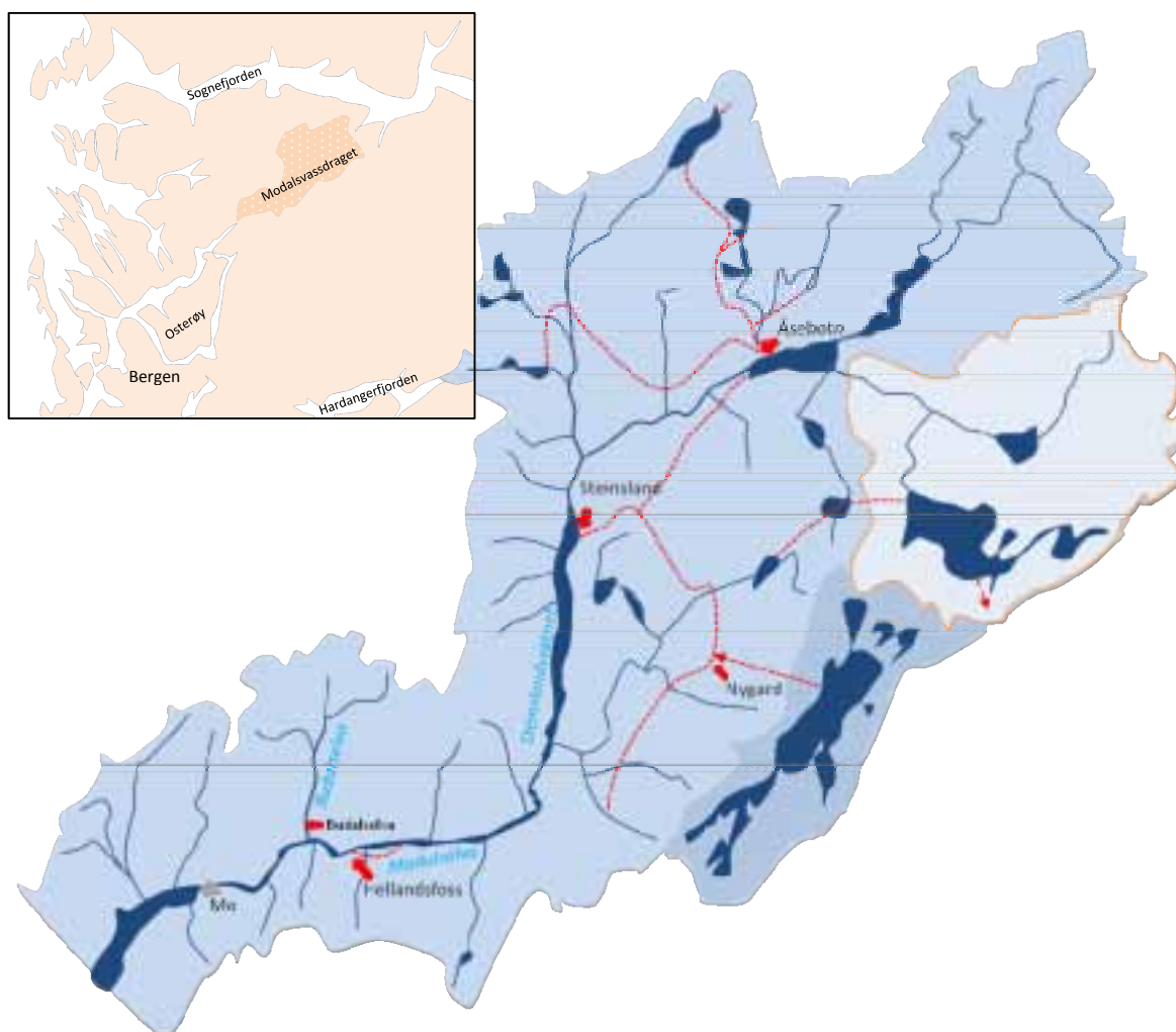
Figur 1. Modalsvassdraget med geografisk beliggenhet. Nedbørsfelt til Modalselva med innsjøer, sidebekker, kraftverk og tunelloverføring av vann. Vann fra de østlige deler av vassdraget blir overført til nabovassdraget.
