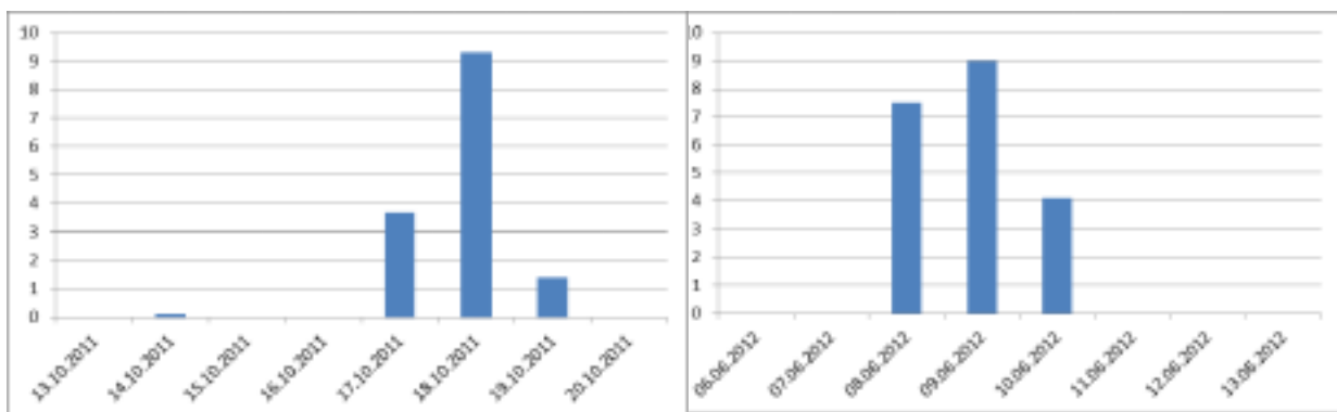
Figur 4. mm nedbør pr døgn i uken forut for prøvetakingene 20.10.2011 og 13.06.2012.
