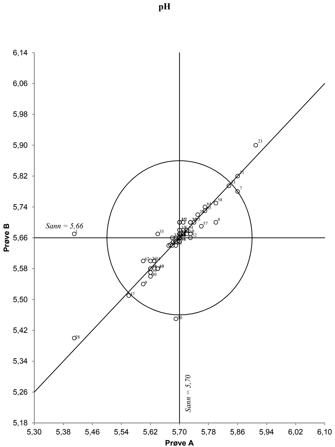
Figur 1. Youdendiagram for pH, prøvepar AB Akseptansegrensen, angitt med en sirkel, er \pm 0,2 pH-enheter
