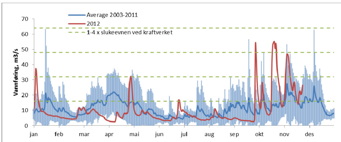
Figur 13. Daglig vannføring ved Lundevatn i 2012 (rød strek). Middelverdien ( \pm 1 \text{ SD} ) for årene 2003 til 2011 er inkludert som blå strek. Vannføringsnivåene 1, 2, 3 og 4 ganger slukeevnen til kraftverket er vist med grønne stiplede linjer.
