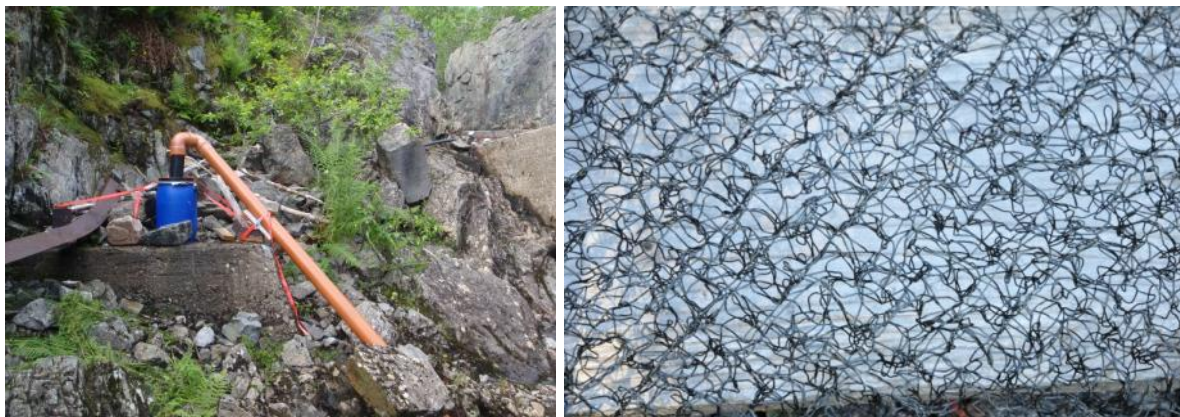
Figur 9. Oppvandringsfelle for ål plassert ved inngangen til nedre laksetrapp ved Fosstveit kraftverk (venstre foto). Enkammat (vevde plasstråder, høyre foto) ble lagt inn i røret for å hjelpe ålen med å vandre opp i fella. Foto: F. Kroglund
