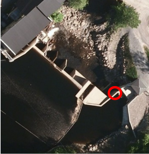
Figur 2. Flyfoto over Fosstveit kraftverk (kilde: Norge i bilder). Slipplokaliteter for PIT-merket ål oppstrøms (rød sirkel) og nedstrøms (gul sirkel) kraftverket, samt og to slipplokaliteter for ål merket med akustiske sendere (blå sirkel) er vist. Selve kraftverksdemningen er forstørret opp nederst. Tiltaksområdet er markert med rød sirkel. En skisse av kaplanturbinen som er installert ved kraftverket er også vist.
