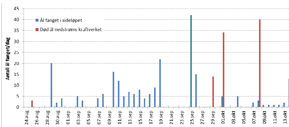
Figur 19. Antall ål som daglig vandret gjennom sideløpet (blå søyler) og antall død ål funnet nedstrøms kraftverket (røde søyler).
