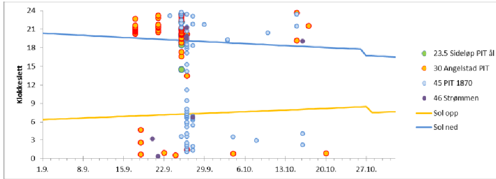
Figur 24. Klokkeslett nedvandrende ål ble påvist på PIT-antenner plassert i vannavskiller ut av sideløpet, ved Angelstad samt ved PIT-1870. De horisontale linjene viser soloppgang og solnedgang. Fiskepasseringene og soloppgang og solnedgang er angitt som GMT+1 (Oslo-tid).
