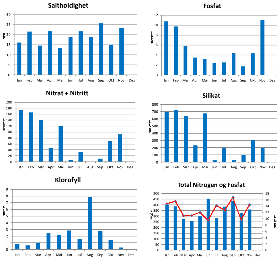
Figur 12. Saltholdighet, Fosfat, Nitrat + Nitritt, silikat, klorofyll a og Total nitrogen og fosfat (sekundær akse, røde punkter) i 2m ved stasjonen "Langesundfjorden" i 2012. Data hentet fra Data hentet fra KLIF-prosjektet "Miljøovervåking av sukkertare".
