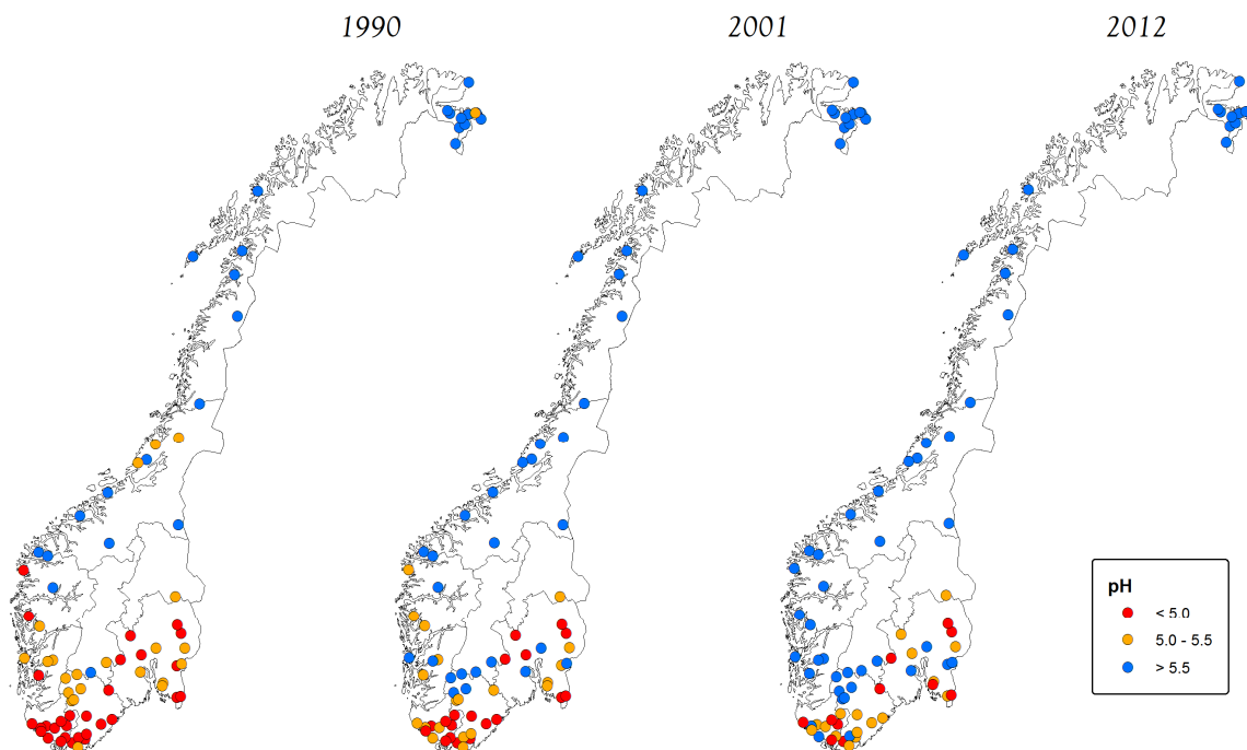
Figur 2. pH i overvåkingsinnsjøene i 1990, 2001 og 2012. Figuren illustrerer tydelig forbedringen i forurensingssituasjonen, ved at sjøene blir mindre sure (får høyere pH). Enkelte sjøer på Østlandet er fortsatt røde, og dette er forårsaket av høyt humusinnhold som gir naturlig lav pH.
