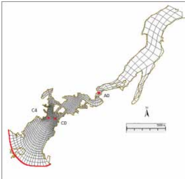
Figur 15. Sandsfjorden ble delt inn i beregningsceller av ulik størrelse. Nær dumpstedet var cellenes horisontale størrelse ca. 50 m x 50 m. I dybderetningen var cellenes utstrekning konstant lik 10 meter. Modellens åpne rand er markert med en rød strek. Tre stasjoner fra modellen er vist som røde prikker.
