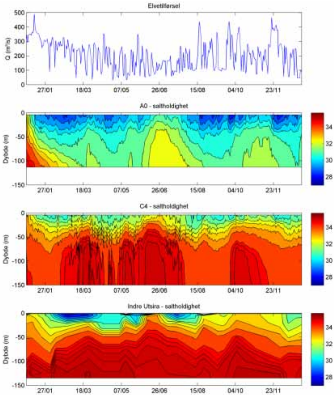
Figur 16. Saltholdigheten på to stasjoner i modellen (A0 og C4) i forhold til indre drivkrefter, vannføringen til fjorden (øverst), og ytre drivkrefter, sjikningen i kyststrømmen (nederst).
