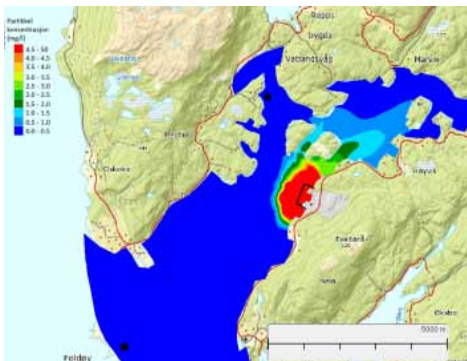
Figur 24. Konsentrasjon av partikler i overflata når det strømmer innover i overflata. Startkonsentrasjonen innenfor den svarte firkanten ved Kvernøysvika var 50 mg/l.
