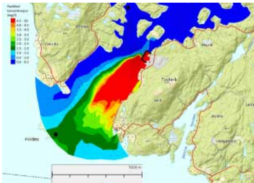
Figur 23. Konsentrasjon av partikler i overflata når det strømmer utover i overflata. Startkonsentrasjonen innenfor den svarte firkanten ved Kvernøysvika var 50 mg/l.
