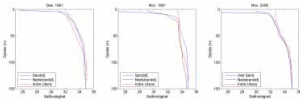
Figur 5. Sammenligning av saltholdighetsprofiler ved stasjon Indre Utsira og Nedstrandfjorden.
