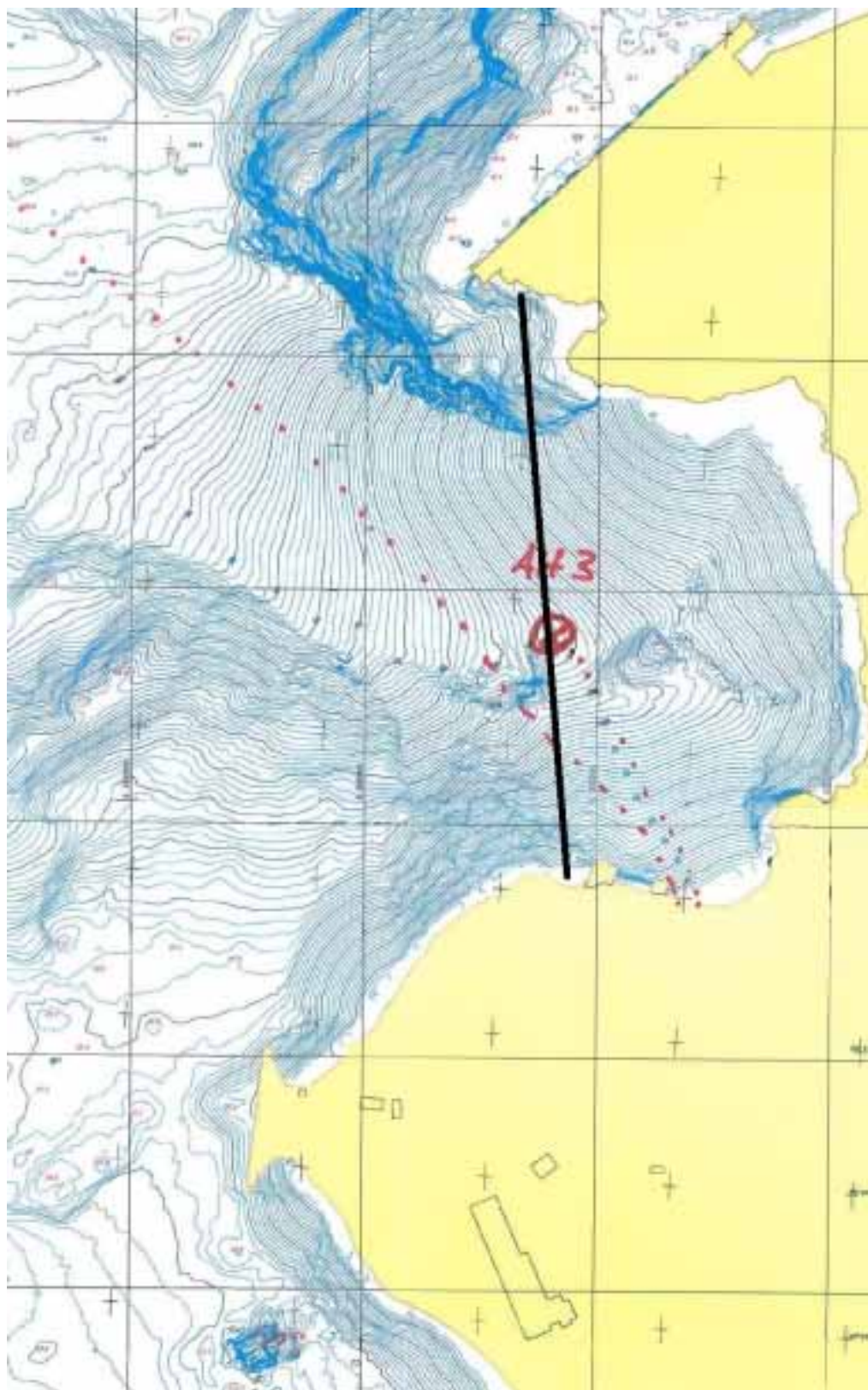
Figur 3. Detaljert bunnkart av Kvednavika (Kilde:Norsk Stein sin utslippsøknad). Siltgardenes omtrentlige plassering er tegnet inn med en tykk svart strek. Størrelsen på rutene er 100 m.
