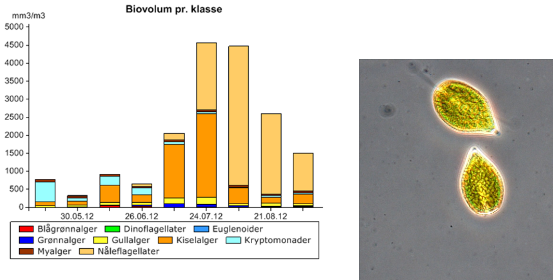
Figur 3. Planteplanktonbiomasse og sammensetning i Sæbyvannet i vekstsesongen 2012. Gonyostomum semen (bildet) tilhører algeklassen Nåleflagellater. Fra Haandes presentasjon på workshopen.
