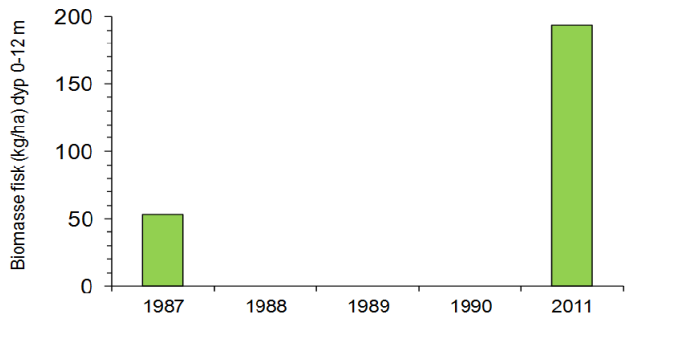
Figur 4. Fiskebiomasse i Sæbyvannet i 2011 sammenlignet med 1987. Brabrand 2012.
