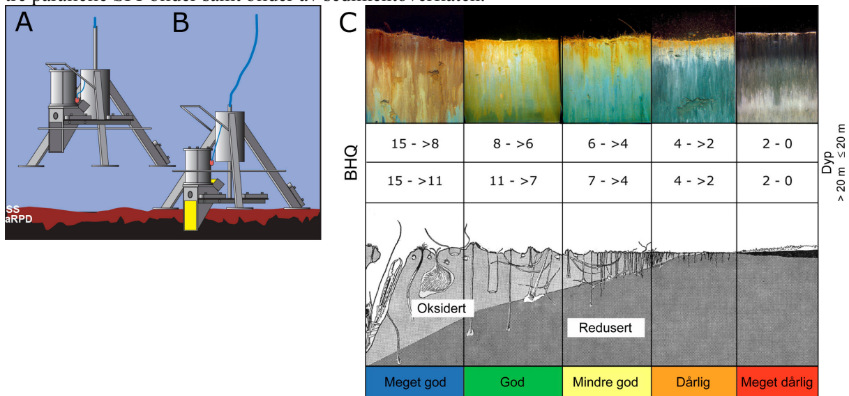
Figur 15. Prinsippskisse for SPI-kamera og bildeanalyse. (A) Kamera og rigg over bunnen (SS = sedimentoverflate og aRPD = grense mellom det bioturberte oksiderte sediment lagret og reduserte sediment [apparent redox potential discontinuity]). (B) Kamera som har trengt ned i sedimentet og bildet eksponeres. (C) Figuren viser endringer i faunatype fra upåvirkede bunnsedimenter med en rik, dyptgravende fauna (Meget god) til en grunnlevende, fattig fauna i påvirkede områder (Meget dårlig). Sedimentprofilbildet er vist i toppen av figuren, der brunt farget sediment indikerer oksidert bioturbert sediment og sorte reduserte forhold. BHQ-miljøkvalitetsindeks for vanddyb \leq 20 meter og > 20 m er i henhold til EUs vanddirektiv for marine sedimenter (Pearson & Rosenberg 1978, Nilsson & Rosenberg 1997, Rosenberg m. fl. 2004, Nilsson & Rosenberg 2006).
