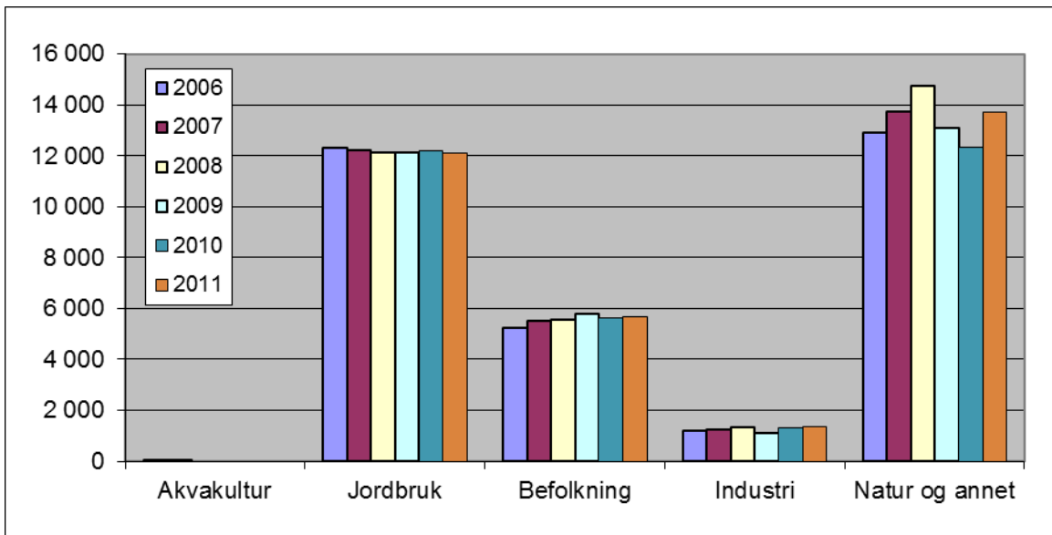
Figur 3. Teoretisk beregnede kildefordelte tilførsler av nitrogen (tonn) til Ytre Oslofjord fra landområdene som drenerer direkte til Ytre Oslofjord. Dette inkluderer avløpsanlegg og industrianlegg med direkte utslipp til fjorden, men tilførsler fra Indre Oslofjord og langtransport med havstrømmene inngår ikke.
