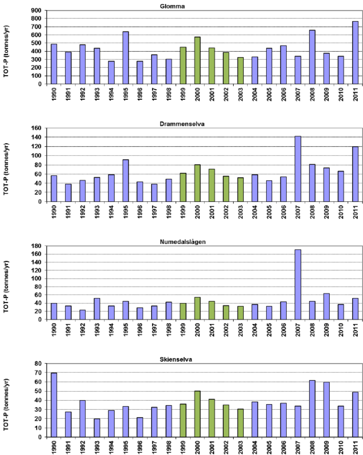
Figur 6. Målte elvetilførsler av total-fosfor i det statlige elvetilførselsprogrammet i perioden 1990 til 2011 (Skarbøvik et al. 2012). År med interpolerte verdier er angitt med grønn farge (målte data fra denne perioden er tatt ut av tidsserien pga. avvikende metodikk).
