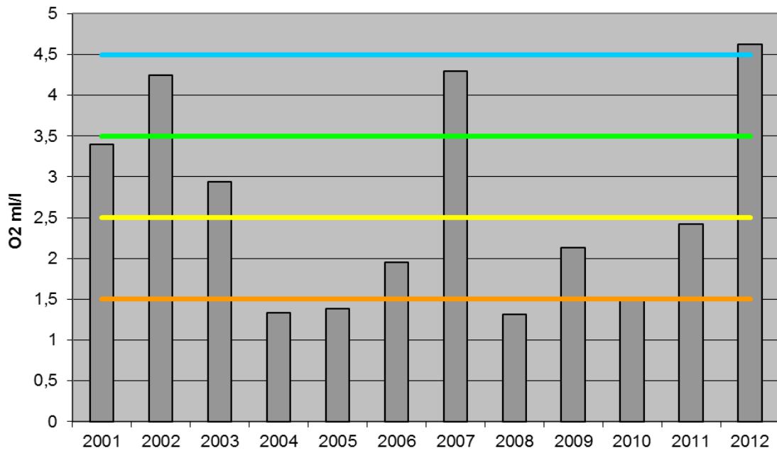
Figur 12. Oksygennivåer i bunnvannet (ca. 30m) i Ringdalsfjorden (RA-5) i september fra 2001 til 2012 (2009-data er fra november). Tilstandsgrensene for SFTs klassifisering av miljøtilstand er indikert i figuren.
