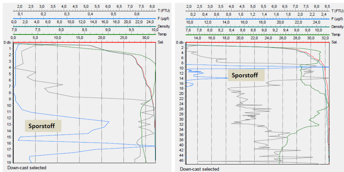
Figur 13. Målte profilar 10. oktober, stasjon 8 (t.v.) og Sta. 29. Sporstoff: Blå kurve, Partiklar/turb.: Svart kurve, Temperatur: Grøn kurve, Salinitet: Raud kurve, Densitet sjøvattn: Grøn kurve.
