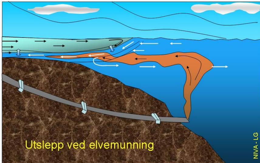
Figur 6. Skisse som viser eit utslepp nær ei elvemunning med ferskvasskile, og korleis utsleppsvatn kan bli transportert i retning inn mot denne.
