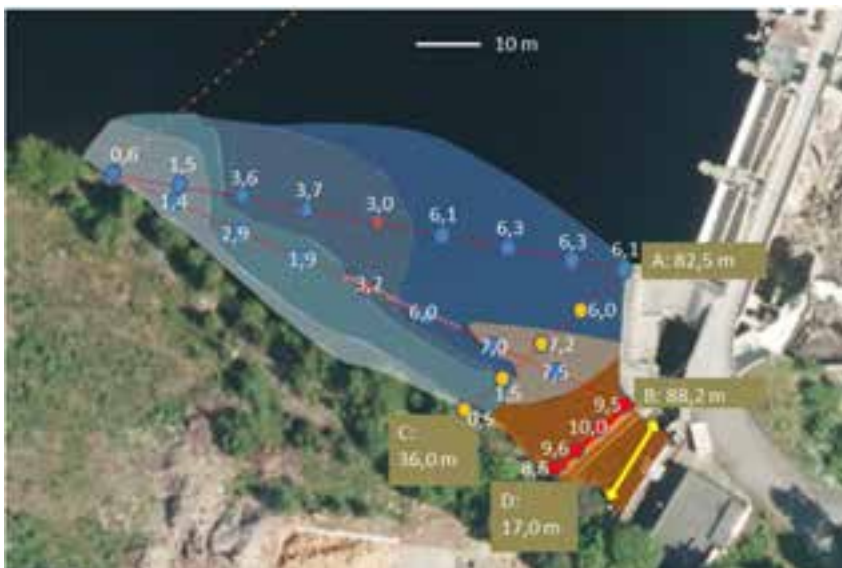
Figur 5. Vanndybder målt langs fire tverrsnitt plassert i inntaksområdet foran Rygene kraftverk. Vanndybdene er deretter illustrert med bruk av fargegradienter.
