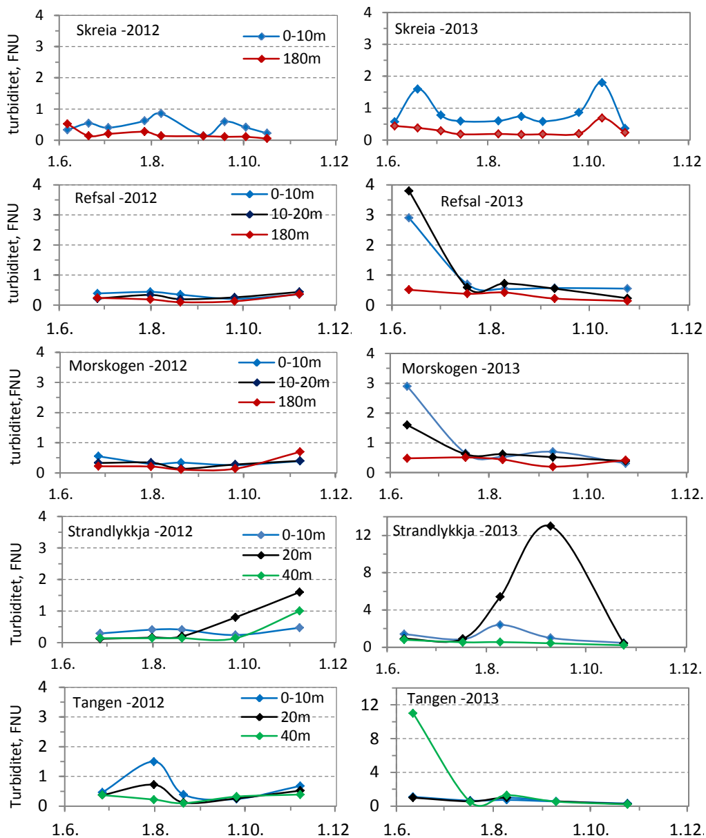
Figur 2. Turbiditeten (FNU) i ulike dyp ved målestasjonene i Mjøsa i 2012 og 2013
