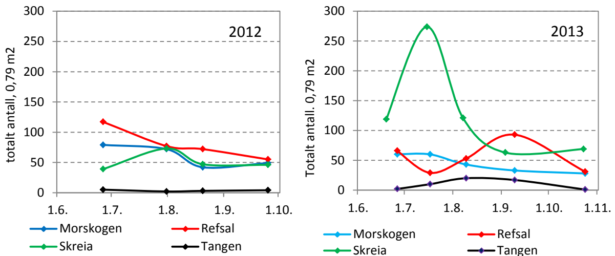
Figur 10. Totalt antall (summen av 0+, 1+ og 2+) av pungreken, Mysis relicta , under 0,79 m 2 fra 0 til 110 m fra slutten av juni til september/oktober.
