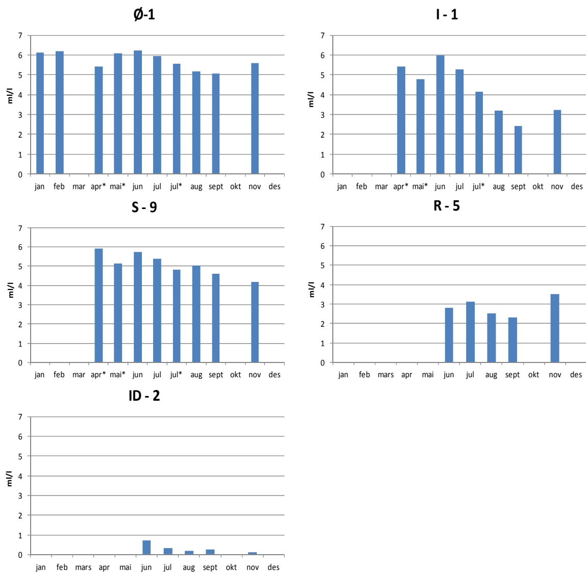
Figur 13. Oksygen - konsentrasjon i dypeste dyp ved stasjonene i Hvaler (Leira Ø-1, Ramsø I-1, Haslau S-9, Ringdalsfjorden RA-5, Iddefjorden ID-2) i 2013. Måned merket med "*" er ekstra prøvetaking for Borregaard AS.
