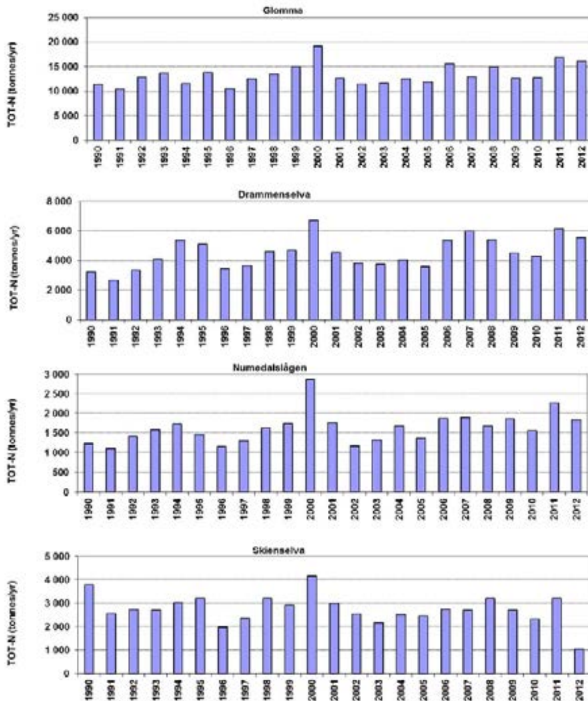
Figur 7. Tilførsler av total nitrogen fra fire elver i perioden 1990-2012 (sakset fra Skarbøvik m. fl. 2013). Lave tilførsler via Skienselva i 2012 er beheftet med usikkerhet pga. en feil som nylig er funnet i vannføringsdata.
