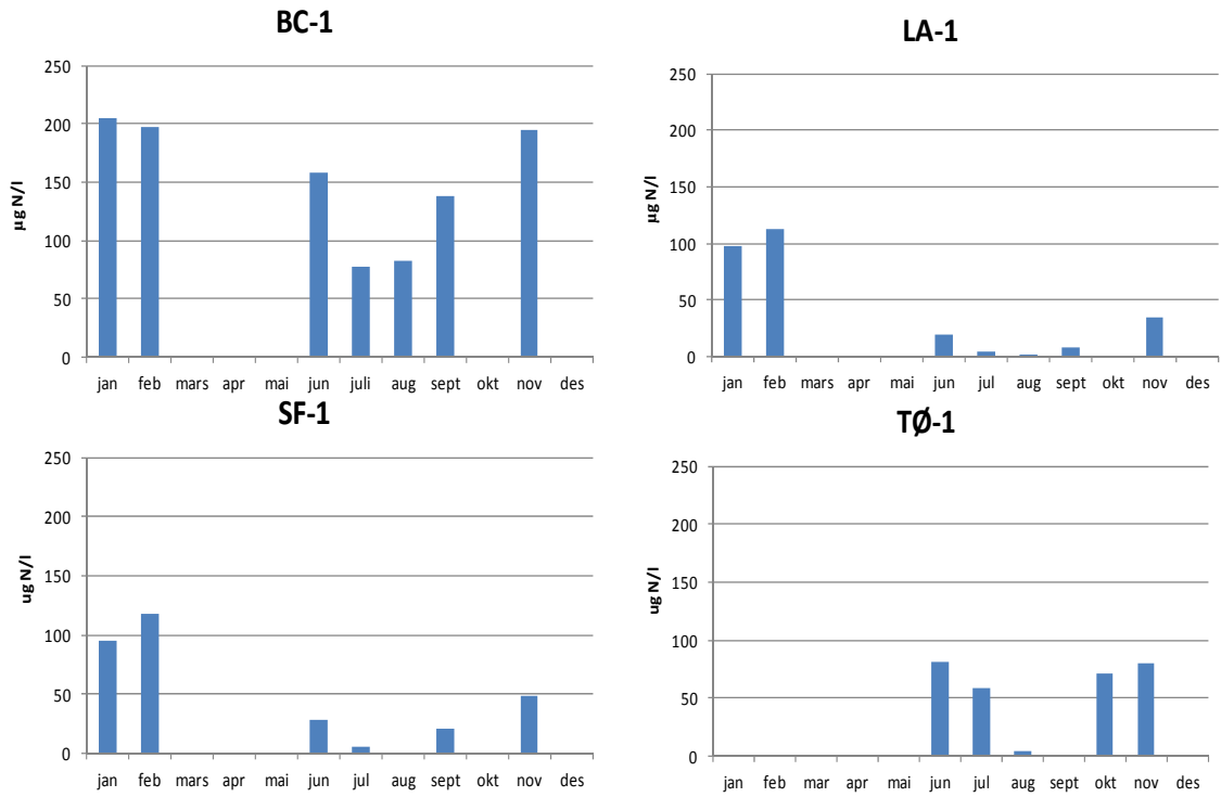
Figur 8. Nitrat + Nitritt-konsentrasjon ( \mu\text{g N/l} ) ved de vestlige stasjonene av Ytre Oslofjord (Larviksfjorden LA-1, Sandefjordsfjorden SF-1, Vestfjorden TØ-1) samt Grenland (Frierfjorden BC-1) i 2013.
